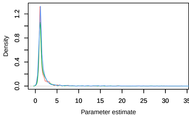
Density – beta_angles[3]
