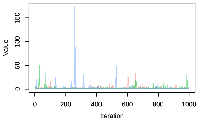
Trace – beta_angles[3]
