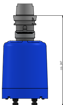
Cloche avec porte-outil HSK-A63
