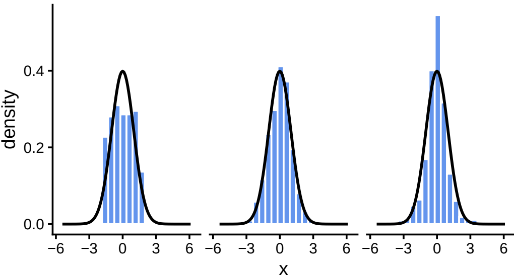
Platykurtic ("too flat")
