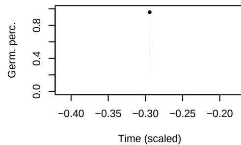
Achillea_erba-rotta, Prov: 79, Chill: -0.44
