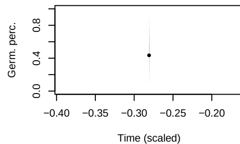
Achillea_erba-rotta, Prov: 83, Chill: -0.44
