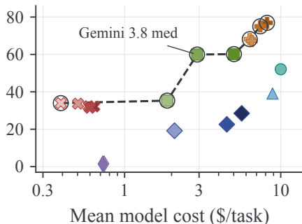
(d) OSWorld2: cost
