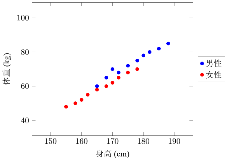
身高与体重关系散点图
