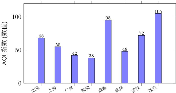
全国主要城市空气质量对比 (AQI 指数)
