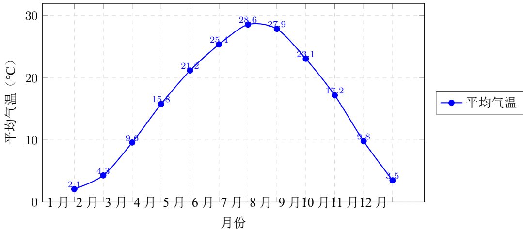
1—12 月平均气温变化趋势
