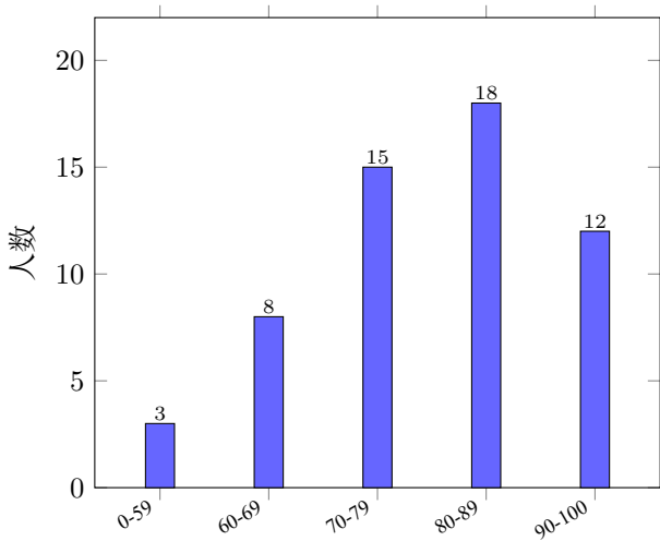
某班成绩分数段人数分布
