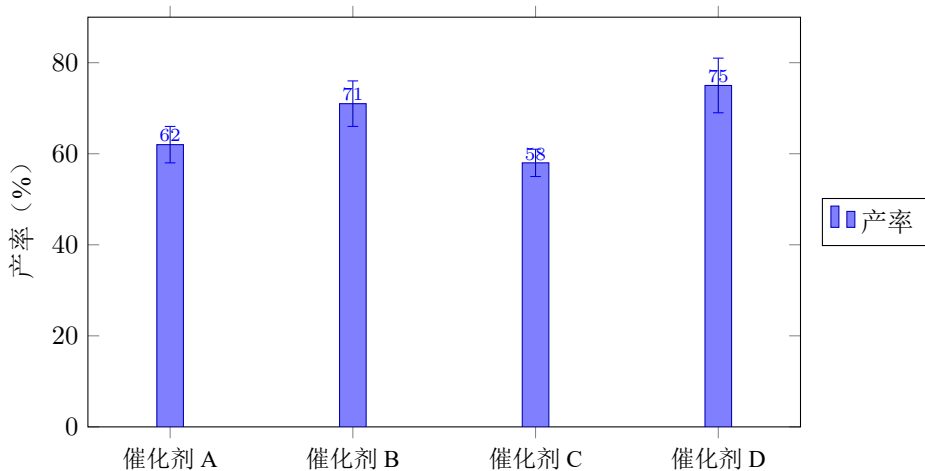
2023 年四种新型催化剂反应产率对比（含标准差误差棒）
