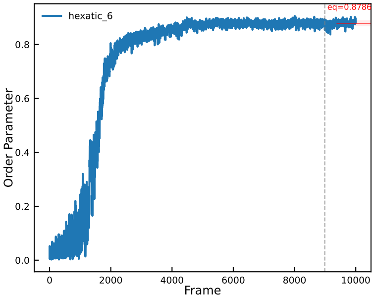
Order Parameters for disk_0
