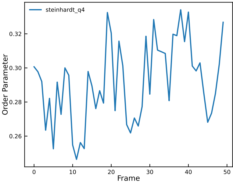
Order Parameters for cube_0
