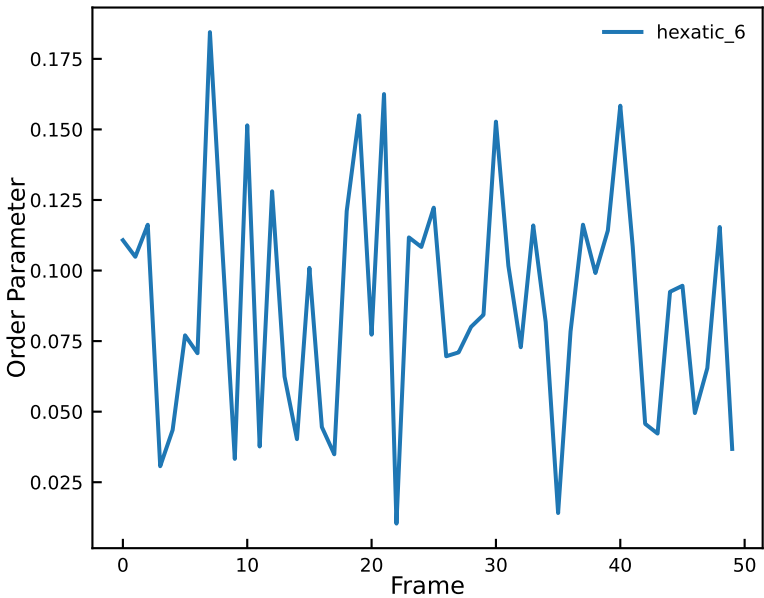
Order Parameters for disk_1
