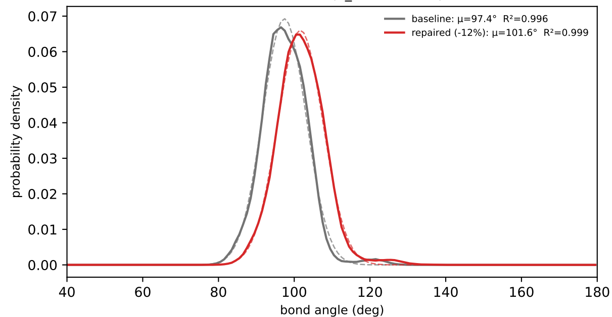
SC1-TN5a-TP2a (n_obs=500020)
