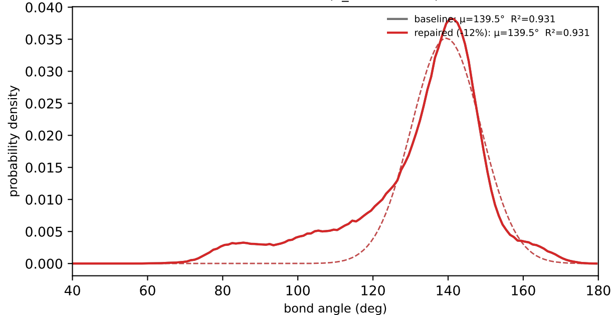
SC1-TN5a-TP2a (n_obs=500020)
