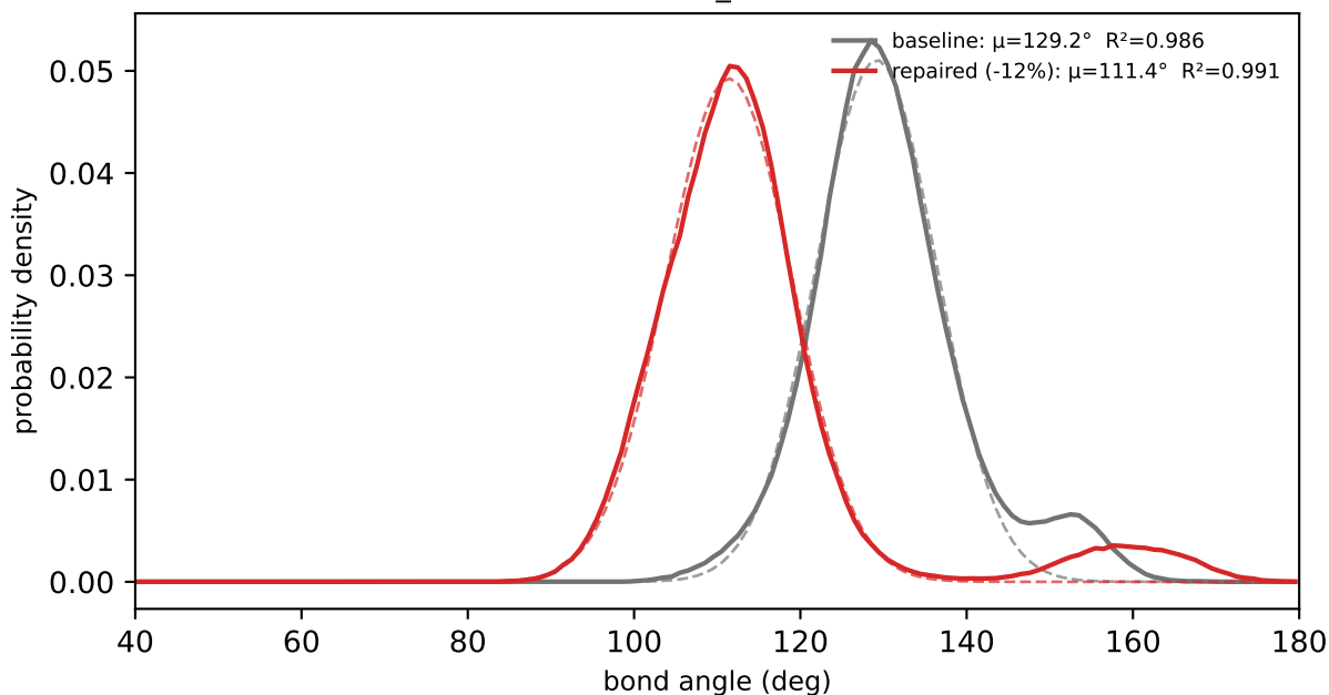
SC1-Q1-TP2a (n_obs=500020)
