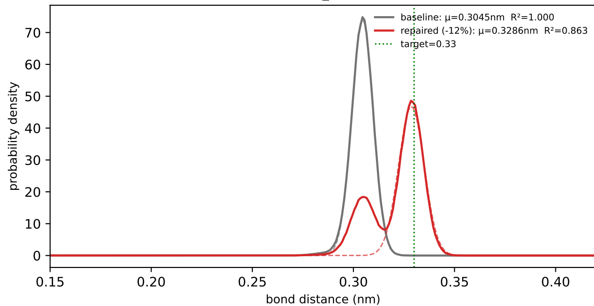
Q1-SC1 #2 (n_obs=500020)
