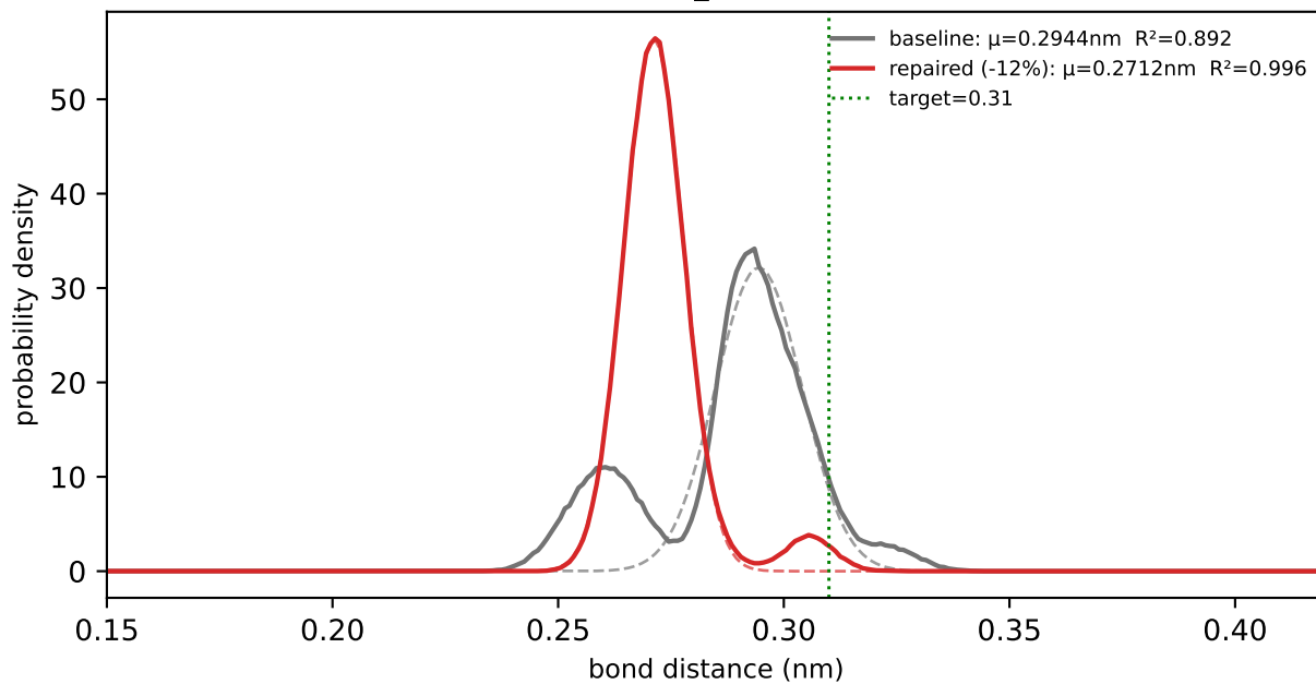
Q1-TP2a (n_obs=500020)
