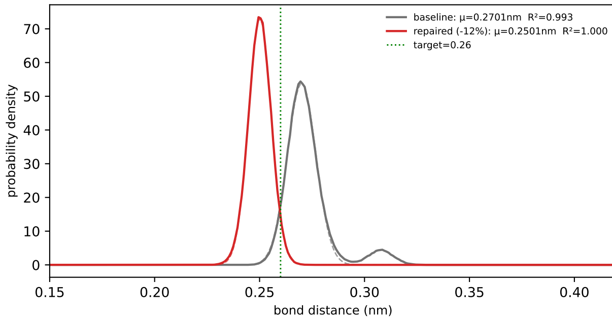
Q1-TP2a (n_obs=500020)
