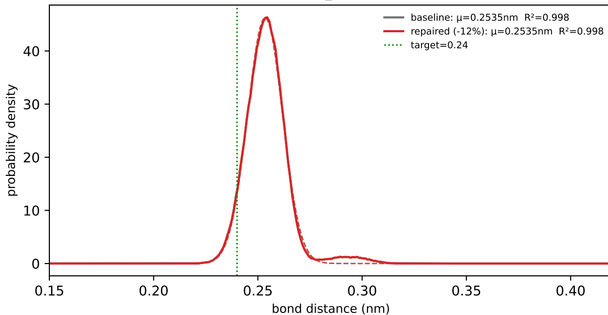
Q1-SC1 #1 (n_obs=500020)
