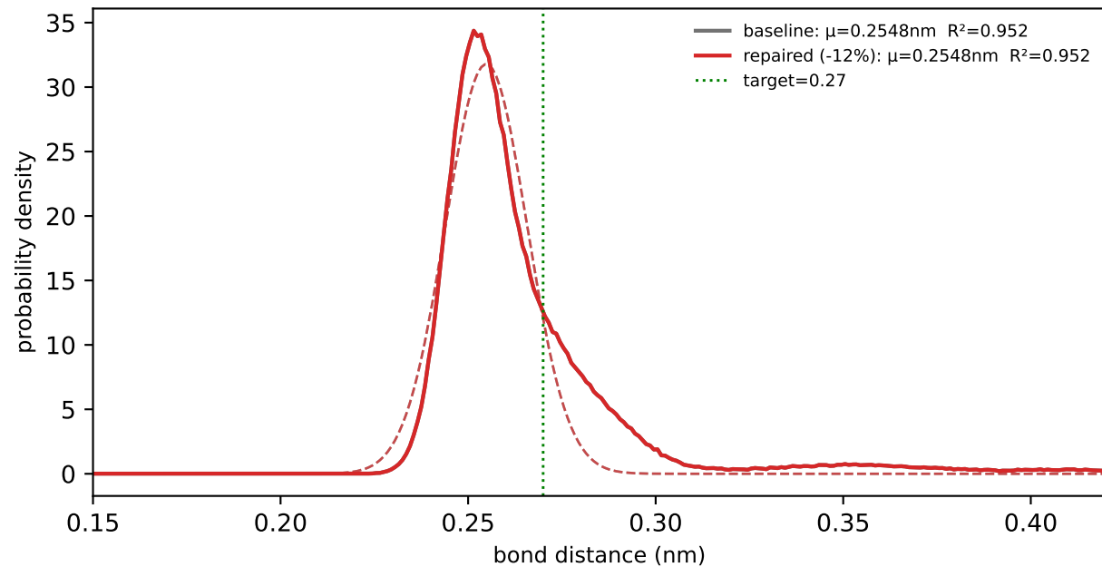
Q1-SC1 #2 (n_obs=500020)
