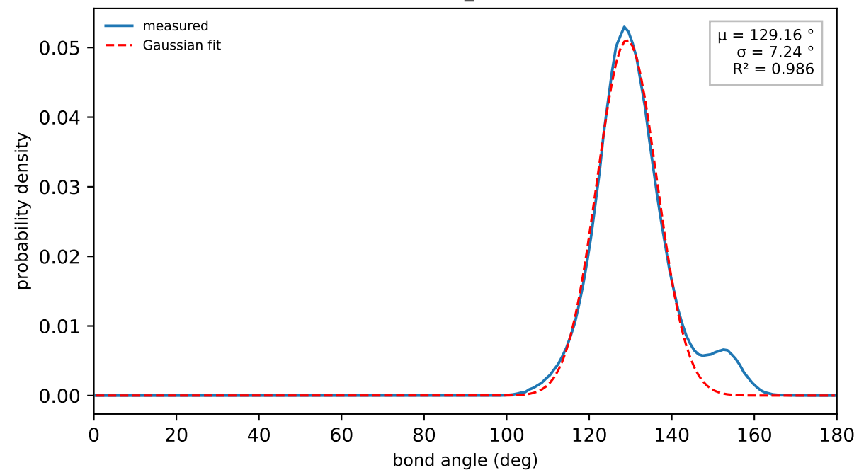
SC1-Q1-TP2a (n_obs=500020)
