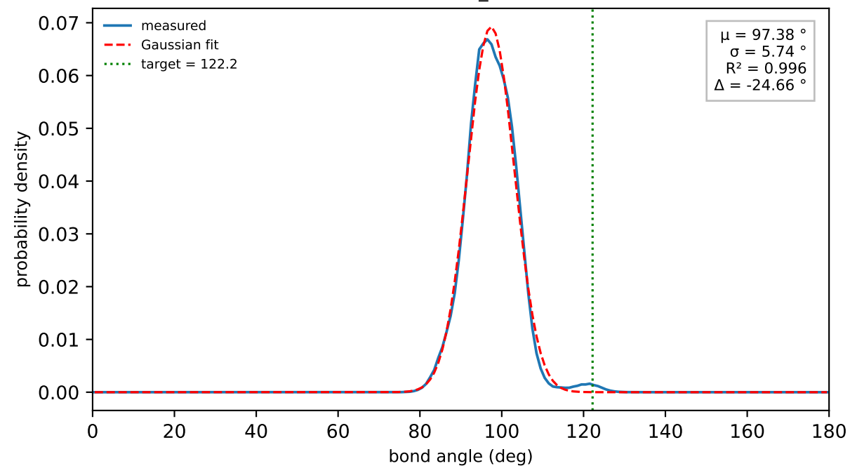
Q1-TP2a-TN5a (n_obs=500020)
