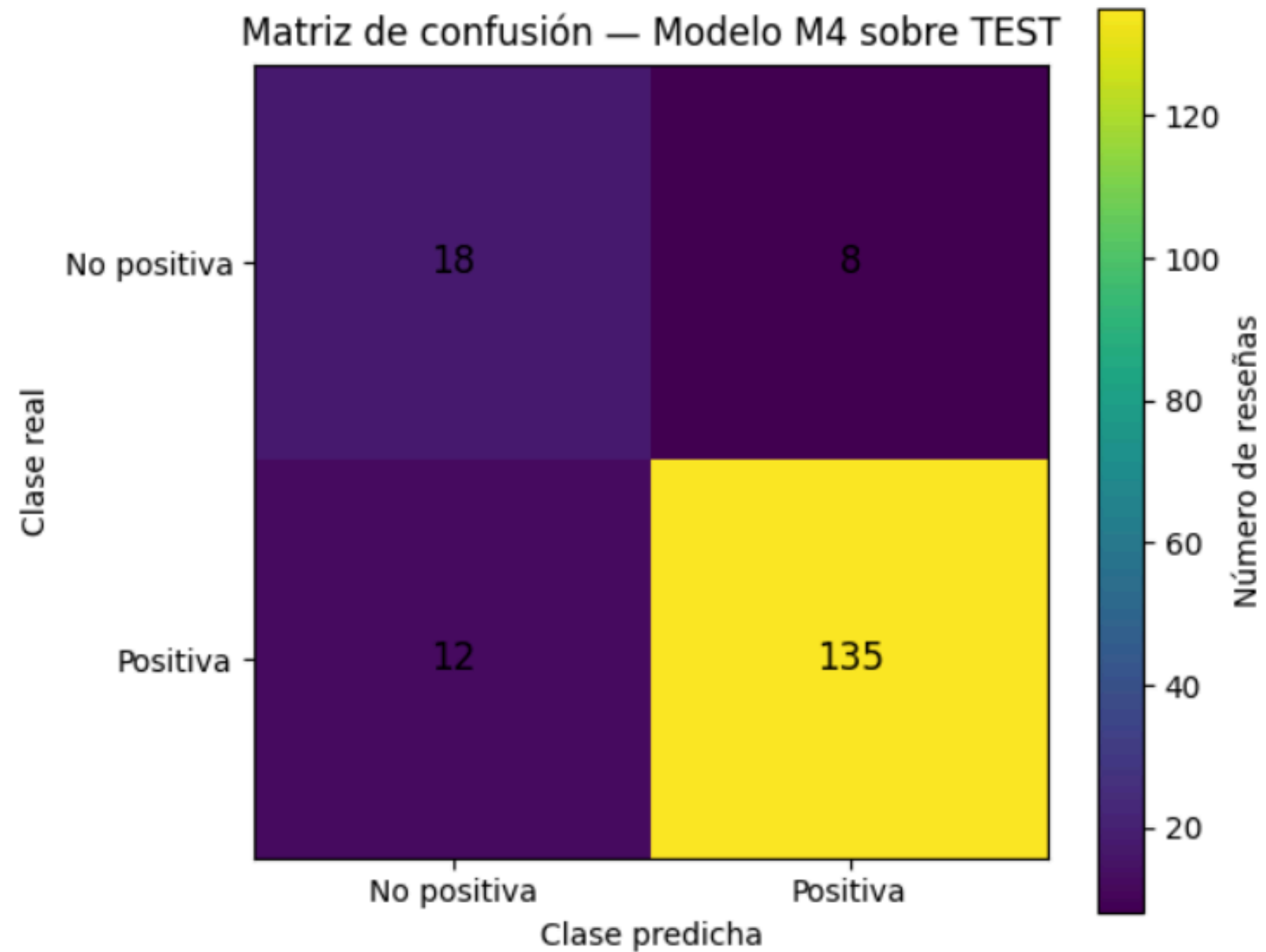
FIGURA 3 – MATRIZ DE CONFUSIÓN TEST
