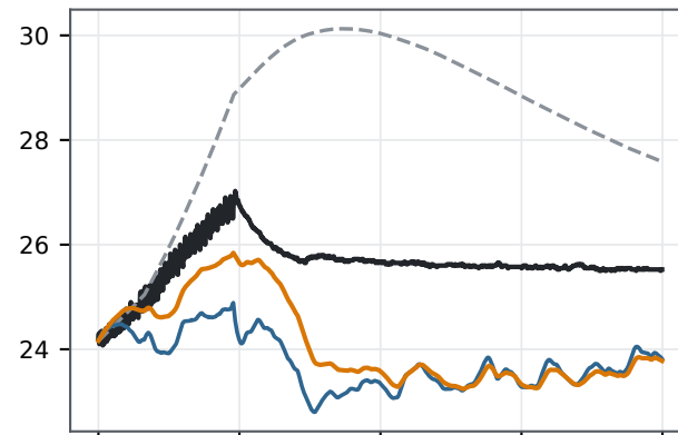
Rotor temperature (°C)
