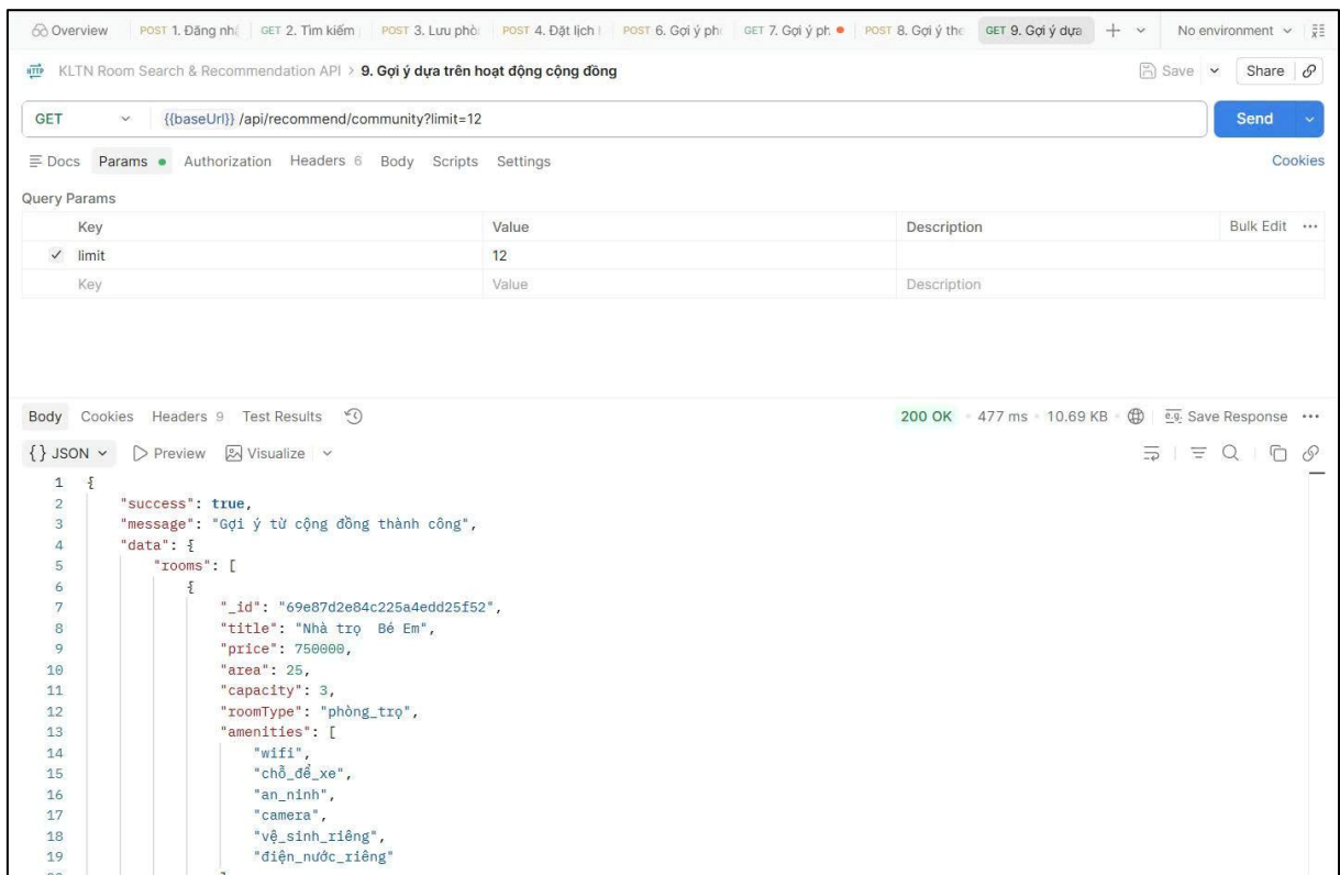
Hình 4.17. Kiểm thử API Gợi ý dựa trên hoạt động cộng đồng bằng Postman
