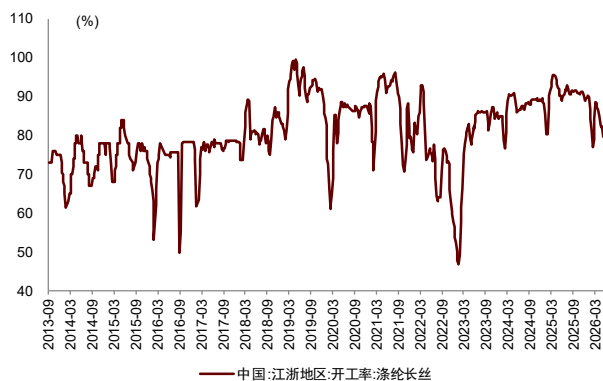
图表 23：生产：涤纶长丝开工率
