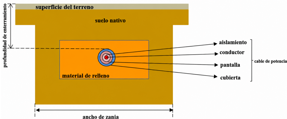
Figura 4.3: Zanja y entorno térmico del cable enterrado: suelo de relleno, suelo nativo, profundidad de instalación y capas principales del cable. Fuente: Enescu et al. (2021:fig. 1).
