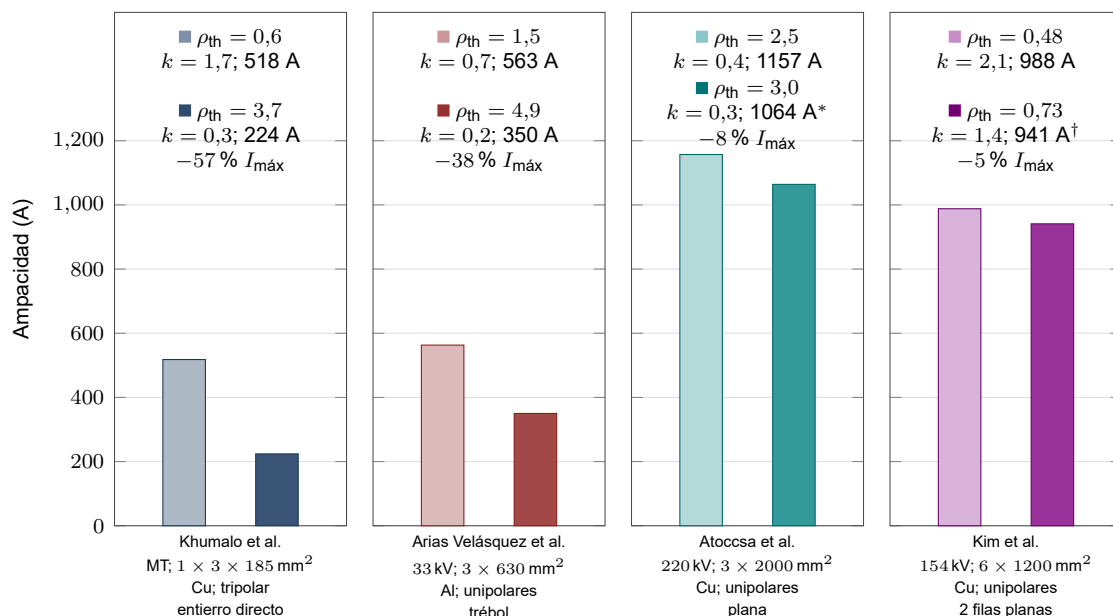
Figura 1.3: Cambio de ampacidad entre dos valores de resistividad térmica en cuatro instalaciones diferentes. Nota: la conductividad térmica es la inversa de la resistividad, k = 1/\rho_{th} ; en las etiquetas, \rho_{th} se expresa en K m/W y k en W/(m K). *Aproximación local de sensibilidad. †Valor leído aproximadamente de la Figura 15 de la fuente, para septiembre y una temperatura del terreno de 21 °C. Fuente: Elaboración propia con datos de Khumalo et al. (2025:5–6, tabs. 2–3), Arias Velasquez et al. (2023:7–8), Atoccsa et al. (2024:15–16) y Kim et al. (2025:4,12–13, fig. 15).
