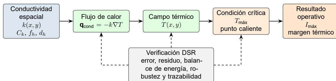
Figura 4.1: Cadena física y metodológica entre heterogeneidad térmica, campo de temperatura y ampacidad. Fuente: Elaboración propia.
