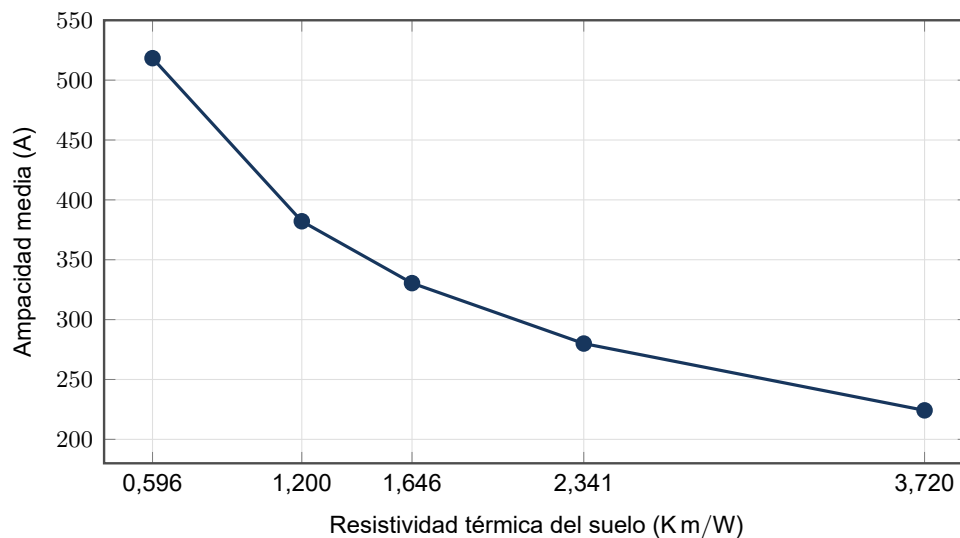
Figura 1.2: Relación entre resistividad térmica del suelo y ampacidad media calculada para tres cables. Fuente: Elaboración propia con datos de Khumalo et al. (2025:5–6, tabs. 2–3).
