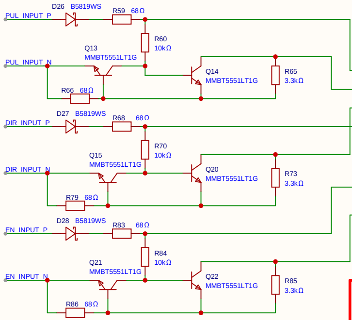
脉冲控制输入信号
