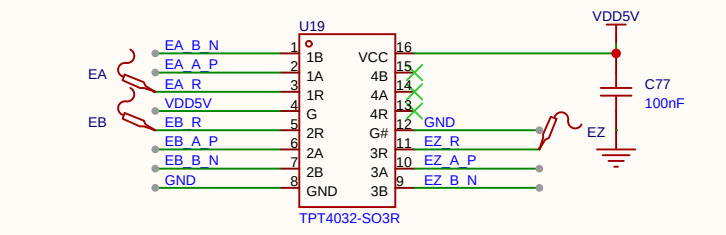
编码器ABZ相输入信号
