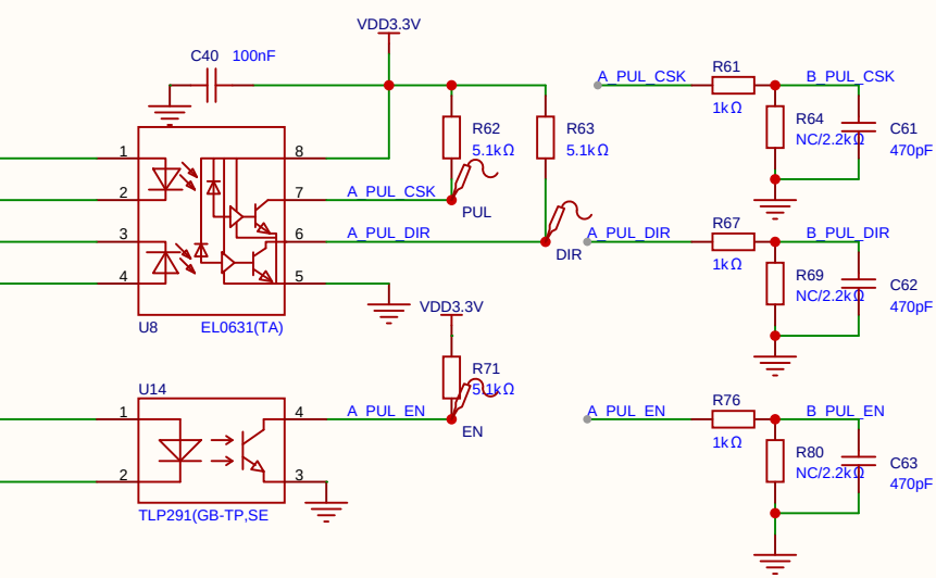
脉冲控制接口
