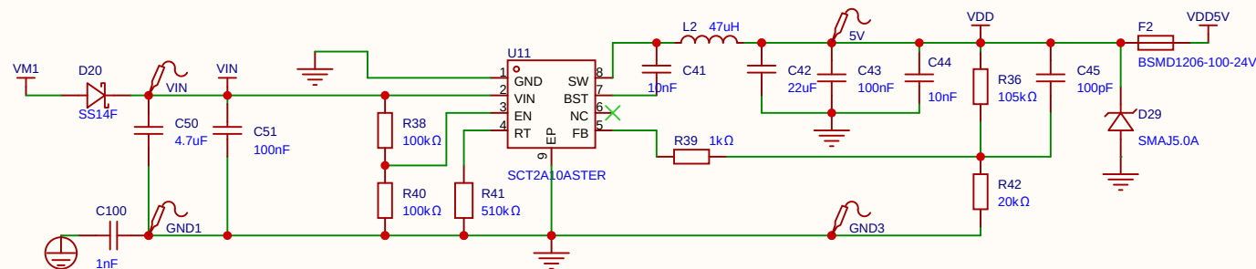
DC-DC转5V电源
