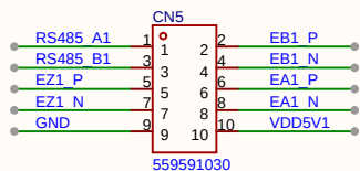
ABZ编码器接口
