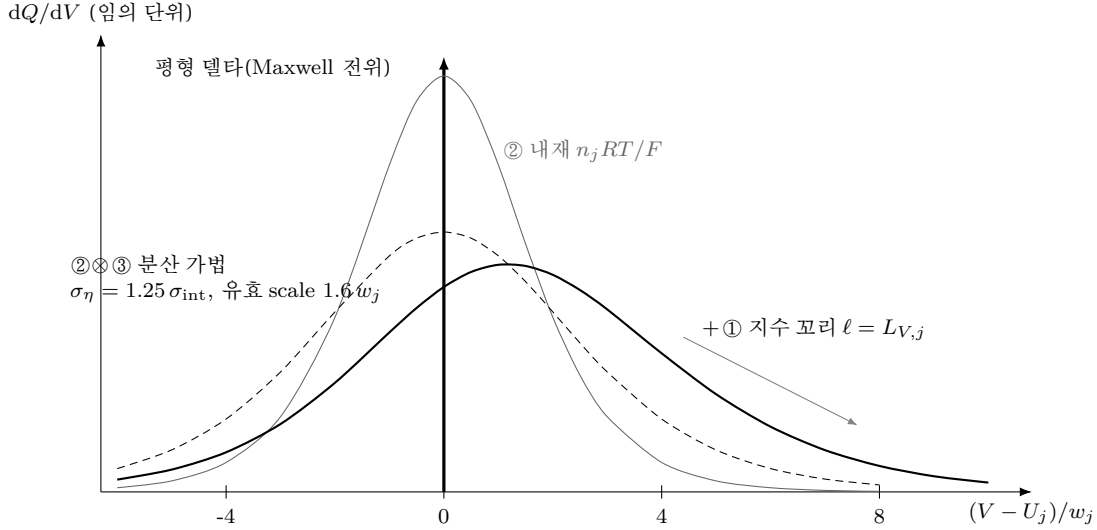
Figure 12: 두-상 broadening 의 폭 예산(식 (1.59); 좌표는 식 그대로의 수치 평가). 평형 델타(수직 화살)에 ② 내재 logistic 미분 중(폭 w_j , 가는 실선)이 없히고, ③ 양상불 \eta 산포와의 합성곱이 분산 가법으로 종을 넓히며(예시 — \eta 산포의 표준편차를 내재 몫의 1.25 배로 두면 \sigma_{\text{sym}} = \sqrt{1 + 1.25^2} \sigma_{\text{int}} \approx 1.6 \sigma_{\text{int}} , 같은 함수족이면 유효 scale 1.6w_j — 파선으로 표시), ① 유한율속이 한쪽 지수 꼬리(예시 L_V = 1.5w_j 와의 단층 합성곱 — 수치 적분)를 늘려 종을 소인 방향으로 민다(굵은 실선). 대칭 두 몫은 w_j 하나에 흡수되고 비대칭 꼬리만 L_{V,j} 로 분리된다.
