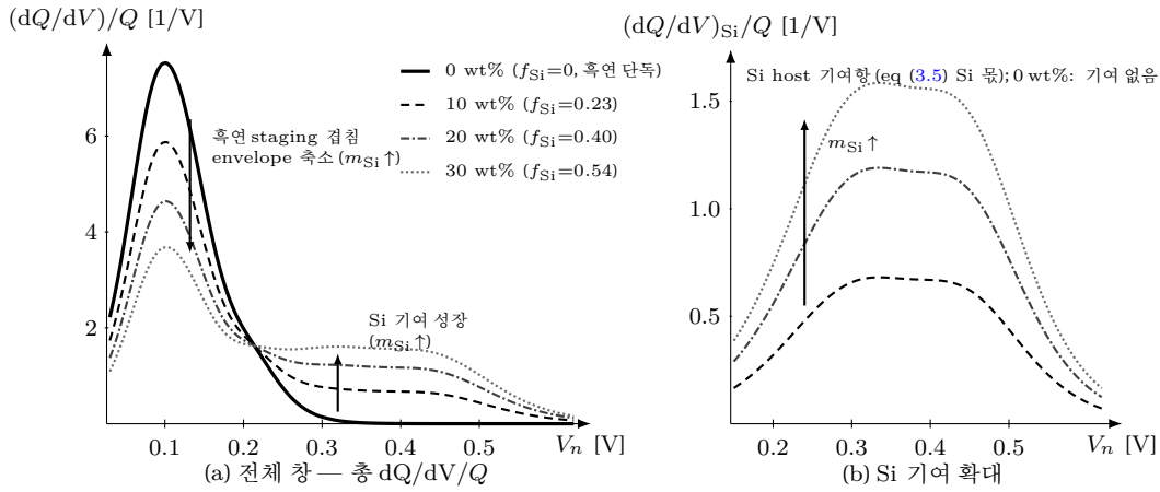
Figure 2: 블렌드 f_{\text{Si}} (wt% 스위치) 가족 평형 dQ/dV — 좌표는 코드 BlendedAnodeDQDV.from_wt(m Si , si_case='elemental') 의 실제산이다: 평형식 (3.5) 의 |I| \rightarrow 0 중 \sum_{\text{host}} \sum_j Q_j^{\text{host}} \xi_{\text{eq},j}^{\text{host}} (1 - \xi_{\text{eq},j}^{\text{host}})/w_j^{\text{host}} 을 T=298.15 \text{ K} , C_{\text{bg}}=0 에서 평가하고 총용량 Q=Q_{\text{gr}}+Q_{\text{Si}} 로 정규화했다(곡선 아래 면적 = 1 규약, 곡선당 ~53–66 표본점). 질량↔용량 환산은 §3.3.1 각주의 환산 규약 f_{\text{Si}} = m_{\text{Si}}q_{\text{Si}}/[m_{\text{Si}}q_{\text{Si}} + (1-m_{\text{Si}})q_{\text{gr}}] ( q_{\text{Si}}=1000 \text{ mAh/g} 원소 Si 1차 가역[2], tier-A· q_{\text{gr}}=372 ) 로, m_{\text{Si}}=0/10/20/30 \text{ wt\%} \Rightarrow f_{\text{Si}}=0/0.230/0.402/0.535 ( Q=0.97/1.26/1.62/2.09 Q_{\text{cell}} ). (a) 전체 창: 흑연 staging 4-peak 겹침 envelope 는 m_{\text{Si}} 증가로 정규화 높이가 7.5 \rightarrow 3.7 [1/V] 로 축소하고( Q_{\text{gr}} 절대값은 불변이나 총용량 Q 가 커져 상대 몫 1-f_{\text{Si}} 로 줄어듦), 원소 Si 두 경사 전이(중심 0.30/0.45 \text{ V} , 폭 0.060/0.050 \text{ V} )의 기여가 고전위 쪽에서 성장해 V_n \approx 0.26 \text{ V} 부근에서 순서가 역전한다. (b) 그 Si host 몫만 떼어(코드 host_contributions ) 확대: 0 \rightarrow 1.585 [1/V] 로 자란다( f_{\text{Si}} 에 정비례). 곡선 개형(전이 중심·폭)은 원소 Si 평균 전위대 0.2\text{--}0.5 \text{ V} [10](tier-B) 안의 tier-C 시연값이며(신뢰값 아님, 피팅 override 전제), elemental 케이스는 \text{SiO}_x 절대전위 같은 “확인 필요” 공백을 쓰지 않는다. f_{\text{Si}} \rightarrow 0 에서 (a)의 실선은 흑연 단독 평형곡선과 부동소수점까지 일치한다(bit-exact, 식 (3.4) 의 코드판; §1.10 그림 18 와 동일 흑연 골격).
