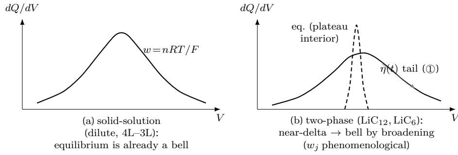
Figure 9: 평형 모양과 broadening(신규). (a) 연속 고용체 전이 — 평형 단일 입자 dQ/dV 가 이미 폭 n_j RT/F 의 중(식 (1.41)), broadening 불요. (b) 2상 전이 — 평형은 plateau 내부에서 거의 날카로운 선(파선, 단 양끝 단상 꼬리 탓에 폭이 정확히 0 은 아님)이나, 실측은 세 출처가 펼친 치우친 종(실선)이다: ① 전류가 켜는 유한율속 비대칭 꼬리(한 입자 안에서 진행 중 변하는 과전압 \eta(t) , §1.9 의 L_V , |I| \rightarrow 0 소멸), ② 전류 무관한 가장자리 내재 폭( \sim RT/F ), ③ 입자 앙상블의 집합 통계역학 — Dreyer 순차 전환이 plateau(평형 델타)를 만들고(평형 층), 그 델타를 펴는 것은 겉보기 중심 U_{app} = U_j + \eta 의 입자간 \eta 산포 \rho(U_{app}) 를 forward 평균한 broadening 층이다(식 (1.42); 비-크기 \eta 산포, 흑연 두-상에 한함). ①의 \eta(t) (한 입자 시간 변화)와 ③의 입자간 \eta 산포는 같은 과전압의 다른 평균이다. 평형 중심 U_j 자체는 입자 무관 상수다 — 분포하는 것은 \eta . 그 폭 w_j 는 평형 예측이 아니라 이 broadening 이 정하는 현상학적 자유 피팅 폭이며, 이 중에서 \rho(U_{app}) 를 역산하거나 입자 사이즈(반경)로 해석하지 않는다(§1.7.2(c)).
