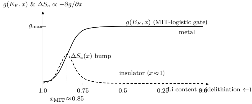
Figure 8: LCO 전자 엔트로피의 MIT-logistic 게이트(신규). 실선 = g(E_F, x) (식 (1.38)): x \approx 1 절연체에서 \approx 0 , 탈리튬화로 x_{MIT} \approx 0.85 부근에서 metal 의 g_{max} = 13 \text{ e/eV} 로 켜진다. 파선 = 탈리튬화 시 방출되는 부분몰 전자 엔트로피 |\Delta S_e| = -\partial S_e / \partial x \propto -\partial g / \partial x > 0 (식 (1.34)·닫힌식 (1.39); 삽입 기준 \Delta S_e = \partial S_e / \partial x < 0 의 절댓값으로, x_{MIT} 에서 \sigma(1 - \sigma) 가 최대): 천이 중심의 국소 봉우리다 — 작지만(O3 부분몰 \approx 0.18 k_B/\text{atom} ) MIT 구간에만 켜지는 게이트라 config 단독으로 대체 불가. \Delta S_{e,j} \propto T 라 다른 항과 달리 전자 기여의 \partial U / \partial T 가 T 에 선형 (§1.6.2; U-이동은 \propto T^2 ). 흑연엔 이 봉우리가 없다( g(E_F) 변화 미미).
