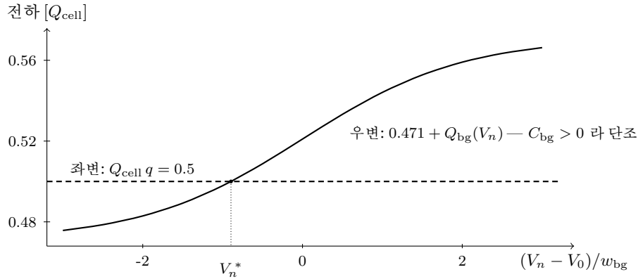
Figure 7: 보존식 (1.42) 의 V_n 결정 — worked example 수치. 우변(실선)이 식 (1.44) 의 단조성으로 좌변(파선)과 한 번 만나는 교점 V_n^* ( Q_{bg} = 0.029 Q_{cell} )가 내부 전위다.
