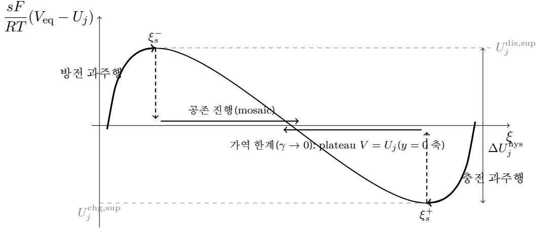
Figure 8: 비단조 평형 전위 (1.66) ( \Omega_j = 4RT )와 과주행 경로. 방전(굵은 경로, 좌상)은 상승 준안정 가지를 타고 극대 \xi_s^- 까지 과주행한 뒤, 분리가 점화되며 공존 plateau ( V = U_j, y = 0 축)로 낙하해 (점선 화살표) mosaic 공존으로 진행한다. 충전(우하)은 거울상으로 극소 \xi_s^+ 까지 과주행한다. 두 극값의 차가 spinodal 상한 gap \Delta U_j^{\text{hys}} 이고(위첨자 sup 는 spinodal 상한 표시), 실측 분기는 축소 인자 \gamma_j 만큼 그 안쪽에 선다 — \gamma \rightarrow 0 의 가역 한계에서 두 경로가 모두 y = 0 의 plateau 로 합쳐진다.
