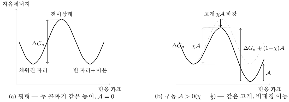
Figure 1: 활성화 장벽 그림(실계산: f_0(x) 이중 골짜기에 구동 기울임 -\mathcal{A}s(x) 를 더한 것, \mathcal{A} = 0.39 \Delta G_a ). (a) 평형 — 두 골짜기가 같은 높이이고 사건 속도는 고개 높이 \Delta G_a 의 Boltzmann 인자에 시도 빈도 k_0 를 곱한 식 (1.1) 을 따른다. (b) 구동력 \mathcal{A}_j 가 도착 골짜기를 \mathcal{A} 만큼 내리면 같은 고개를 공유하는 두 방향의 장벽이 비대칭으로 변한다 — 정방향은 \Delta G_a - \chi\mathcal{A} 로 낮아지고 역방향은 \Delta G_a + (1 - \chi)\mathcal{A} 로 높아진다 (§1.4 식 (1.15) 의 시각 짝; 점선은 (a)의 평형 풍경). 온도는 풍경을 기울이지 않는 대신 지수의 분모( RT )로 들어와 넘는 확률 자체를 키운다(고개 높이의 엔트로피 몫 -T\Delta S_a 는 §1.10 의 절편으로 처리된다).
