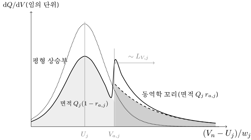
Figure 6: 닫힌식 (1.61) 한 전이의 해부( r_{a,j} = 0.315 , L_V = 3w ). 점선은 평형 종(기준선), 파선은 동역학 꼬리, 실선이 닫힌식의 합이다. 상승부 실선이 점선보다 낮은 간격이 종 항의 (1 - r_{a,j}) 인자 — 꼬리로 넘어간 미완 몫의 회계 — 이고, 열은 음영(종 성분)과 진한 음영(꼬리 성분)의 면적이 각각 Q_j(1 - r_{a,j}) 와 Q_j r_{a,j} , 합이 정확히 Q_j 다(식 (1.62)의 시각 짝). 꼬리는 V_{a,j} 에서 진폭 r_{a,j}/L_{V,j} 로 점화되어 단방향으로만 살며, 점화 계단은 지시함수의 모델 성질이라 r_{a,j} 가 클수록 크고 실측에서는 평활이 뭉갸다. 점화점이 U_j + 2.2w 에 놓인 것은 본 그림의 합성 조건에서 q -축 5% 컷이 맞히는 V -축 상(像)이라서다 — |dV/dq| 압축 때문에 V -축의 평형 종은 그 점에서 아직 유한하다.
