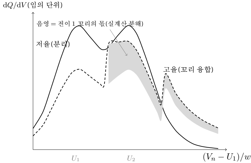
Figure 7: 두 인접 전이의 융합(중심 간격 3.9w ). 실선은 저울( r_a \rightarrow 0 ) — 골이 깊어 분리가 일어난다. 파선은 고울( r_a = 0.35 , L_V = 4w ) — 식 (1.64) 그대로, 중 항이 (1 - r_a) = 0.65 로 깎이고 각 전이의 꼬리가 다음 전이 쪽으로 뻗어 골의 우측을 매우고 뒤 어깨를 들어 올리므로 분리 판독이 지워진다. 음영 때가 그 주변 — 고울 곡선에서 전이 1 꼬리가 보태는 뭉(실계산 분해: 진폭 r_a/L_V = 0.0875 의 지수) — 이며, 골 위와 전이 2의 어깨 위에 걸쳐 있는 것이 보인다. 저온도 같은 방향으로 작용한다.
