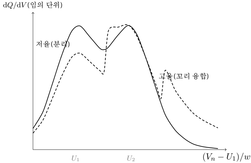
Figure 5: 두 인접 전이의 융합 모식(중심 간격 3.9w ). 실선은 저울 — 두 peak 사이 골이 깊어 분리가 쉽다. 파선은 고울 — 각 전이의 동역학 꼬리( L_V = 4w )가 다음 전이 쪽으로 뻗어 골을 매우 고 뒤쪽 어깨를 들어 올리며, 면적이 섞이기 시작한다. 저온도 같은 방향으로 작용한다(꼬리 길이 \propto |I|e^{\Delta H_a/RT} ). 융합 후의 식별은 §1.10의 forward 합산만 허용된다.
