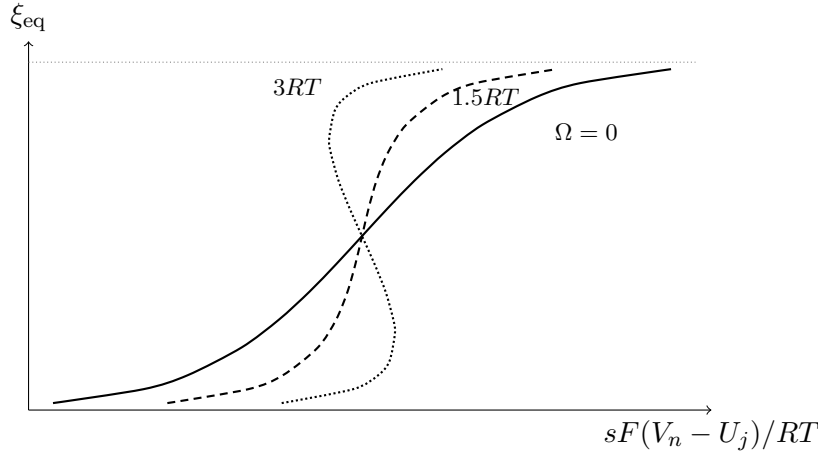
Figure 2: 평형 등온선의 한 모수축. 이상( \Omega = 0 , 실선)은 폭 RT/F 의 logistic, \Omega = 1.5RT (파선)는 같은 함수축이되 중심 기울기가 가팔라진(좁아진) 단조 곡선, \Omega = 3RT > 2RT (점선)는 비단조가 되어 한 전위에 세 \xi 가 대응하는 다가구간이 생긴다 — 그 다가성이 §1.12 분기의 뿌리다.
