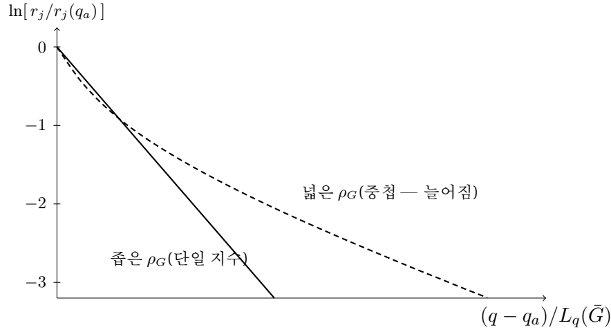
Figure 4: 지수 감쇠의 연속 중첩(반로그). 실선은 단일 배리어(좁은 \rho_G )의 순수 지수 — 반로그에서 직선이다. 파선은 감쇠 길이 L/3 , L , 3L 세 집단을 같은 무게로 섞은 중첩 — 초기엔 빠른 집단이 끌어들여 가파르고, 후미에선 느린 집단만 남아 완만해진다. 이 “직선에서 아래로 휘는” 모양이 stretched 꼬리의 지문이며, 피팅 알고리즘의 잔차 진단 (§1.16)에서 \rho_G 적분을 켜는 신호다.
