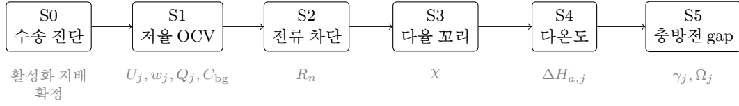
Figure 9: 비순환 식별 사슬 S0→S5. 각 단계의 출력(아래 라벨)은 다음 단계에서 동결된 기지값으로 쓰이므로, 단계마다 미지수가 하나씩만 남아 공선형이 끊긴다. 화살표를 거슬러 자유화하는 것은 금지된다.
