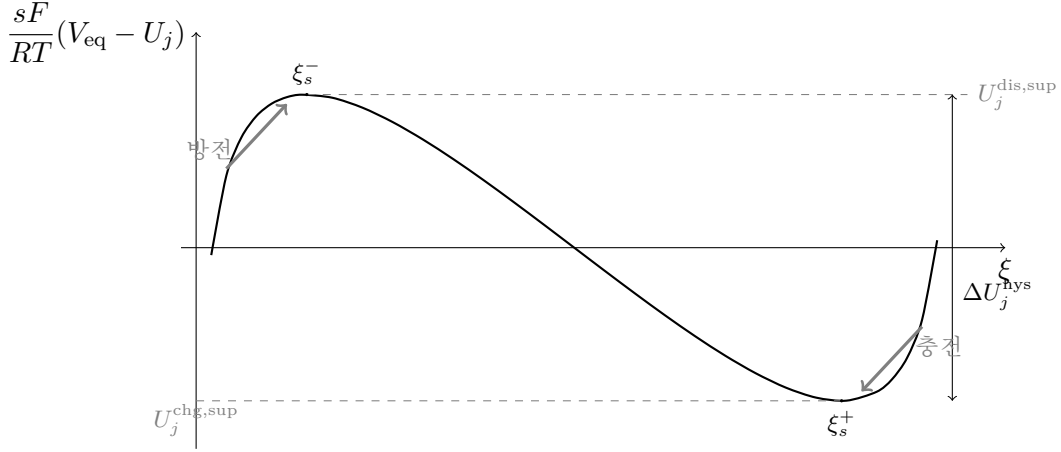
Figure 6: 비단조 평형 전위 V_{eq,j}(\xi) ( \Omega_j = 4RT , 식 (1.44)). 방전은 \xi \approx 0 에서 출발해 상승 준안정 가지를 타고 극대 \xi_s^- 까지, 충전은 반대쪽 \xi_s^+ 까지 과주행한다. 두 극값의 전위 차가 spinodal 상한 gap \Delta U_j^{\text{hys}} (식 (1.48)) 이고, 실측 분기는 축소 인자 \gamma_j 만큼 그 안쪽에 선다(식 (1.49)).
