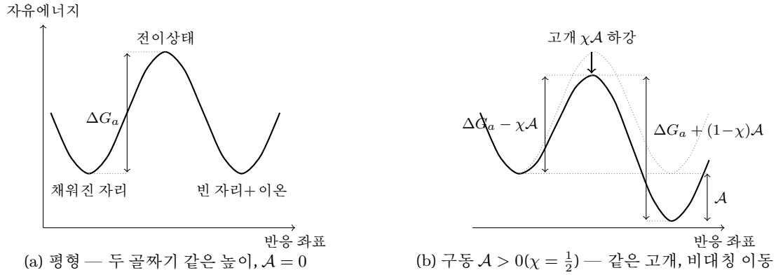
Figure 2: 활성화 장벽 그림(실계산: f_0(x) 이중 골짜기에 구동 기울임 -As(x) 를 더한 것, A = 0.39 \Delta G_a ). (a) 평형 — 두 골짜기가 같은 높이이고 사건 속도는 고개 높이 \Delta G_a 의 Boltzmann 인자에 시도 빈도 k_0 를 곱한 식 (1.1)을 따른다. (b) 구동력 A_j 가 도착 골짜기를 A 만큼 내리면 같은 고개를 공유하는 두 방향의 장벽이 비대칭으로 변한다 — 정방향은 \Delta G_a - \chi A 로 낮아지고 역방향은 \Delta G_a + (1 - \chi)A 로 높아진다 (§1.4 식 (1.15)의 시각 짝; 점선은 (a)의 평형 풍경). 온도는 풍경을 기울이지 않는 대신 지수의 분모( RT )로 들어와 넘는 확률 자체를 키운다(고개 높이의 엔트로피 몫 -T\Delta S_a 는 §1.10의 절편으로 처리된다).
