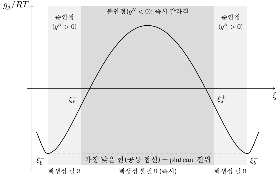
Figure 4: 가운데가 언덕이 된 자유에너지( \Omega_j = 3RT — 곡선은 식 (1.26), 띠 경계는 식 (1.28)의 실제 산값). 곡선이 현(파선)보다 위에 있는 두 점점 \xi_b^\pm 사이에서는 갈라지는 쪽이 이득이다 — 이 경계가 binodal 이고, 접선의 기울기가 plateau 전위다. 진한 띠( \xi_s^- < \xi < \xi_s^+ , g'' < 0 )는 미소 요동에도 즉시 무너지는 불안정 영역 — 경계가 spinodal 이다. 옅은 띠(binodal–spinodal 사이)가 준안정 — 갈라지면 이득이지만 핵생성 장벽을 넘어야 도달하는 영역 — 이며, 충방전 히스테리시스의 무대가 된다. 띠 밖(binodal 바깥)은 균질 단상이 최선인 안정 영역이다.
