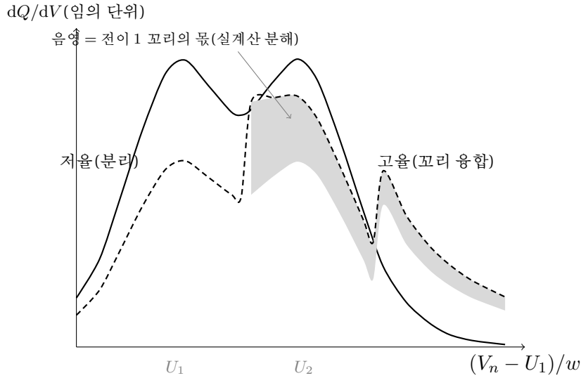
Figure 8: 두 인접 전이의 융합(중심 간격 3.9w ). 실선은 저울( r_a \rightarrow 0 ) — 골이 깊어 분리가 쉽다. 파선은 고울( r_a = 0.35 , L_V = 4w ) — 식 (1.64) 그대로, 중 향이 (1 - r_a) = 0.65 로 깎이고 각 전이의 꼬리가 다음 전이 쪽으로 뻗어 골의 우측을 매우고 뒤 어깨를 들어 올리므로 분리 관독이 지워진다. 음영 때가 그 주변 — 고울 곡선에서 전이 1 꼬리가 보태는 뭉(실계산 분해: 진폭 r_a/L_V = 0.0875 의 지수) — 이며, 골 위와 전이 2 의 어깨 위에 걸쳐 있는 것이 보인다. 저온도 같은 방향으로 작용한다.
