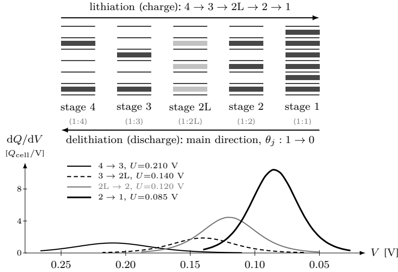
Figure 2: 흑연 staging 의 갤러리 채움 도식(위)과 대응 dQ/dV peak(아래, 식 (1.57) 의 초기값 수치 평가 — dQ/dV = Q_j \xi_{\text{eq}}(1 - \xi_{\text{eq}})/w_j , 표 2 의 U_j, Q_j, w_j ). 위: 수평선이 그려진 층, 음영 띠가 리튬이 든 층간 갤러리다. 채울수록 stage 번호가 줄어 stage 1(LiC 6 , 완전 채움)에 닿고, 열 아래 비율(1:4→1:1) 이 각 stage 의 갤러리 점유 주기다. stage 2L 은 면내 질서가 풀린 단계라 열게 표시했다. 아래: 네 초기값 전이의 실제 peak — 높이 Q_j/(4w_j) 는 전이마다 크게 다르다 ( 2 \rightarrow 1 이 가장 큼, 10.4 Q_{\text{cell}}/V ). 주의 — 위 갤러리 열 간격은 범주형(등간격 스케치)이고 아래 V 축은 실제 전위 스케일(비등간격 — 3 \rightarrow 2L 과 2L \rightarrow 2 은 겨우 20 mV 차이로 갤러리 열 간격에 선형 정렬되지 않는다)이라, 둘은 전이명 (예 2 \rightarrow 1 )으로만 대응시킨다. 본 문건 방향은 방전(탈리튬화)이다.
