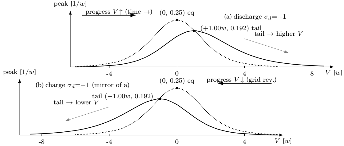
Figure 15: 인과 꼬리의 방향 — 좌표는 저역통과 점화식(식 (1.73))의 수치 평가( w=1 , L_V=1.5w , \rho=e^{-\Delta_{\text{grid}}/L_V}=0.967 ). 점선 = 평형 종 \xi_{\text{eq}}(1-\xi_{\text{eq}})/w (정점 0.25@중심, 방향 불변), 실선 = peak shape (\xi_{\text{eq}}-\xi_{\text{lag}})/L_V (식 (1.74)). (a) 방전은 진행이 V\uparrow 라 꼬리가 높은 V 쪽으로, 정점 (+1.00w, 0.192) (격자 그대로). (b) 충전은 진행이 V\downarrow 라 격자를 뒤집어 필터한 뒤 되돌려(식 (1.76)) 꼬리가 낮은 V 쪽으로, 정점 (-1.00w, 0.192) — 방전의 정확한 거울. 두 경우 모두 peak 는 양수.
