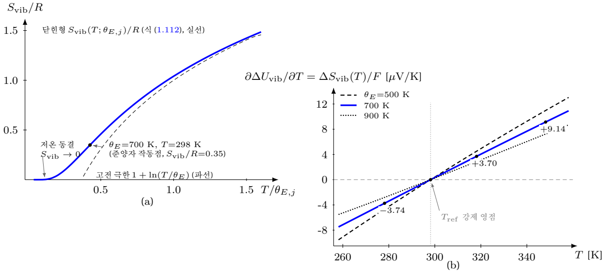
Figure 20: Einstein 진동 보정의 두 얼굴 — 좌표는 식 (1.112)·(1.114) 그대로의 수치 평가다. (a) 단한형 S_{\text{vib}}(T; \theta_{E,j})/R : 저온( u_j \rightarrow \infty )에서 0 으로 동결되고 고전 극한(파선) 1 + \ln(T/\theta_E) 에 T/\theta_E \gtrsim 1 에서 붙는다 — 앞 절이 중심 표준값에 흡수한 “ T -무관 상수”는 이 곡선을 T_{\text{ref}} 에서 한 번 평가해 동결한 값이다. ● 는 \theta_E = 700 \text{ K} · 298 \text{ K} 의 준양자 작동점. (b) 중심 이동의 온도 기울기 \partial \Delta U_{\text{vib}} / \partial T = \Delta S_{\text{vib}}(T)/F : \theta_E = 500/700/900 \text{ K} 모두 T_{\text{ref}} 의 강제 영점을 지나 로그형 곡률로 자라며, ● 는 본문 §1.14.3 의 수치 ( \theta_E = 700 \text{ K} 에서 -3.74/0/+3.70/+9.14 \mu\text{V/K} ) 다. electronic 항( \propto T )은 이 강제 영점이 없어 두 함수형이 다운도 곡률 피팅에서 갈리고, 분리에는 준양자 창을 걸치는 온도점 셋 이상이 필요하다.
