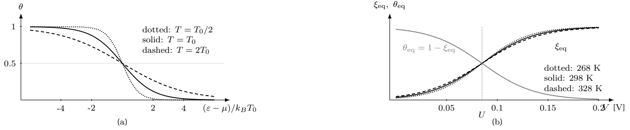
Figure 6: 단일 자리 점유의 전기화학적 재매개변수화(좌표는 식 그대로의 수치 평가). (a) 식 (1.14)의 \theta - \varepsilon = \mu 에서 \frac{1}{2} , 낮은 T 일수록 계단( \beta \rightarrow \infty - T \rightarrow 0 극한이 계단 함수다), 높은 T 일수록 완만. (b) 식 (1.32)의 \xi_{eq}(V) ( U = 0.085 V, stage 2 \rightarrow 1 초기값) — 폭 w = RT/F 가 23.1/25.7/28.3 mV(268/298/328 K)로 T 에 비례해 열리고, 회색 \theta_{eq} = 1 - \xi_{eq} 와 중심 V = U 에서 교차한다( \frac{1}{2} ).
