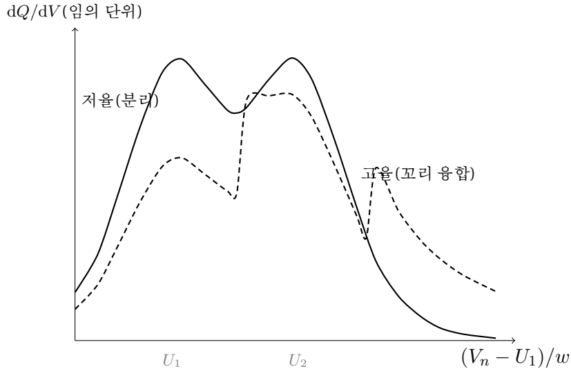
Figure 7: 두 인접 전이의 융합(중심 간격 3.9w ). 실선은 저울( r_a \rightarrow 0 ) — 골이 깊어 분리가 일어난다. 파선은 고울( r_a = 0.35, L_V = 4w ) — 식 (1.58) 그대로, 중 항이 (1 - r_a) = 0.65 로 깎이고 각 전이의 꼬리가 다음 전이 쪽으로 뻗어 골의 우측을 메우고 뒤 어깨를 들어 올리므로 분리 판독이 지워진다. 저온도 같은 방향으로 작용한다.
