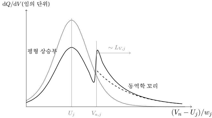
Figure 6: 닫힌식 (1.57) 한 전이의 해부( r_{a,j} = 0.315 , L_V = 3w ). 점선은 평형 중 (기준선), 파선은 동역학 꼬리, 실선이 닫힌식의 합이다. 상승부 실선이 점선보다 낮은 간격이 종 항의 (1 - r_{a,j}) 인자 — 꼬리로 넘어간 미완 몫의 회계 — 다. 꼬리는 V_{a,j} 에서 진폭 r_{a,j}/L_{V,j} 로 점화되어 단방향으로만 살며, 점화 계단은 지시함수의 모델 성질이라 r_{a,j} 가 클수록 크고 실측에서는 평활이 뭉갸다. 점화점이 U_j + 2.2w 에 놓인 것은 본 그림의 합성 조건에서 q -축 5% 컷이 맺히는 V -축 상(像)이라서다 — |dV/dq| 압축 때문에 V -축의 평형 중은 그 점에서 아직 유한하다.
