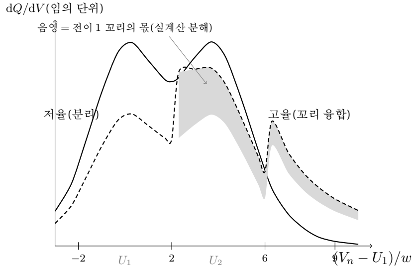
Figure 12: 두 인접 전이의 융합(중심 간격 3.9w ). 실선은 저울( r_a \rightarrow 0 ) — 골이 깊어 분리가 일어난다. 파선은 고울( r_a = 0.35 , L_V = 4w ) — 식 (1.82) 그대로, 중 향이 (1 - r_a) = 0.65 로 깎이고 각 전이의 꼬리가 다음 전이 쪽으로 뺏어 골의 우측을 매우고 뒤 어깨를 들어 올리므로 분리 판독이 지워진다. 음영 때가 그 주변 — 고울 곡선에서 전이 1 꼬리가 보태는 뒀(실계산 분해: 진폭 r_a/L_V = 0.0875 의 지수) — 이며, 골 위와 전이 2의 어깨 위에 걸쳐 있는 것이 보인다. 저온도 같은 방향으로 작용한다.
