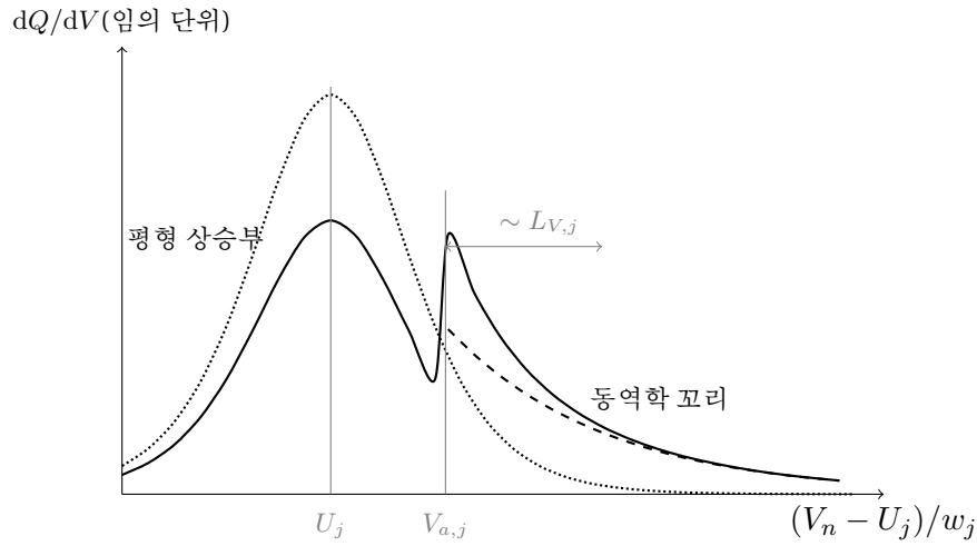
Figure 6: 닫힌식 (1.52) 한 전이의 해부( r_{a,j} = 0.315 , L_V = 3w ). 점선은 평형 중 (기준선), 파선은 동역학 꼬리, 실선이 닫힌식의 합이다. 상승부 실선이 점선보다 낮은 간격이 종 항의 (1 - r_{a,j}) 인자 — 꼬리로 넘어간 미완 몫의 회계 — 다. 꼬리는 V_{a,j} 에서 진폭 r_{a,j}/L_{V,j} 로 점화되어 단방향으로만 살며, 점화 계단은 지시함수의 모델 성질이라 r_{a,j} 가 클수록 크고 실측에서는 평활이 뭉갸다. 점화점이 U_j + 2.2w 에 놓인 것은 본 그림의 합성 조건에서 q -축 5% 컷이 맏히는 V -축 상(像)이라서다 — |dV/dq| 압축 때문에 V -축의 평형 중은 그 점에서 아직 유한하다.
