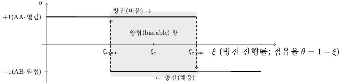
Figure 17: 적층 order parameter \sigma 의 방향별 이력(식 (1.98)–(1.100); \xi_c = 0.5 , \Delta\xi_{\text{stack}} = 0.4 ). 충전 ( \xi 감소, 점유율 증가)은 닫힘( \sigma = -1 )을 유지하다 \xi_{\text{open}} = 0.3 (점유율 70%)에서 열리고, 방전( \xi 증가)은 열림( \sigma = +1 )을 \xi_{\text{close}} = 0.7 (점유율 30%)까지 버티다 닫는다(점선: 점화 점프). 두 임계 조성의 분리가 방향 비대칭이며, 음영의 bistable 창이 그 폭이다. B_j \rightarrow 0 에서 창이 닫혀 §1.13의 대칭 그림으로 회수된다.
