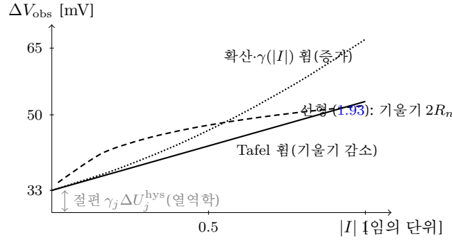
Figure 14: 관측 gap 의 분해 (1.93) (실계산: 절편 33 mV, 기울기 20 mV/단위). 실선이 가산 분해의 예측 — |I| \rightarrow 0 절편이 열역학 같림, 기울기가 분극이다. 파선은 charge-transfer 의 Tafel 휨(기울기 점감), 점선은 확산 한계· \gamma_j(|I|) 의 휨(점증) — 두 휨이 가산 분해 전제의 위반 지문이며 진단표 (§1.15)가 받는다.
