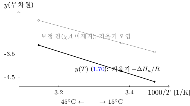
Figure 9: Arrhenius 회귀 (1.71) 의 시각(실계산: \Delta H_a = 40 kJ/mol, 절편 12, 세 온도 15/23/45°C). 검정 점·직선은 보정된 측정량 y(T) (1.70) — 정확히 1/T 에 선형이고 기울기가 -\Delta H_a/R 다. 회색 점은 구동항 \chi A_j/RT 를 빼지 않은 경우( \chi A = 2.9 kJ/mol 예시) — 점이 위로 밀리고 기울기가 오염된다. S4 가 \chi 를 먼저 닫는 이유(§1.15)가 이 그림이다.
