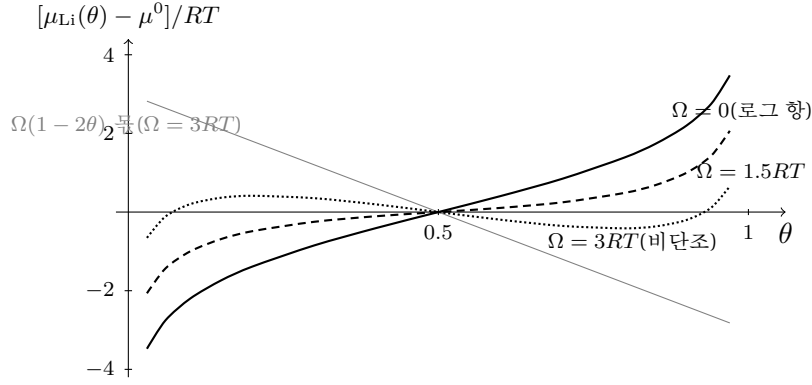
Figure 3: 화학퍼텐셜 (1.13)의 해부(실계산). 실선은 \Omega = 0 의 로그(섞임 엔트로피) 몫 — 채울수록 값어치가 단조로 오른다. 회색 가는 선은 상호작용 몫 \Omega(1-2\theta) ( \Omega = 3RT ) — 반대 기울기의 직선이다. 둘을 더하면: \Omega = 1.5RT (파선)는 가운데가 평평해진 단조 곡선, \Omega = 3RT > 2RT (점선)는 비단조 — 한 값어치에 세 조성이 대응하며, 이것이 상분리의 씨앗이다 (§1.5).
