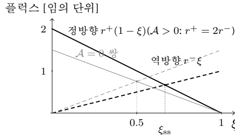
Figure 4: 정지점의 시각화(실계산). 정방향 플럭스 r^+(1-\xi) 는 차 있는 자리가 줄며 감소하는 직선, 역방향 r^-\xi 는 빈 자리가 늘며 증가하는 직선 — 교점이 정지점 (1.25) 이다. A > 0 ( r^+ = 2r^- 예시, 검정 쌍)이면 교점이 \xi_{ss} = 2/3 로 밀리고, A = 0 (회색 쌍)이면 \frac{1}{2} — 구동력이 정지점을 미치는 방식 (1.26) 그 자체다.
