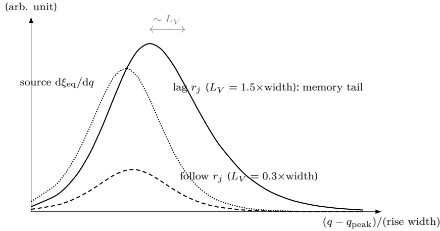
Figure 7: 지연 ODE 일반해 (1.43) 의 두 거동(신규). 점선 = 원천 d\xi_{eq}/dq (중). 파선 ( L_V = 0.3 \times 폭) = 빠른 동역학의 축소 추종(정점 \approx L_V \times 원천, r \rightarrow 0 평형 복귀). 실선 ( L_V = 1.5 \times 폭) = 기억이 상승부를 덮어 정점이 늦고 높으며, 원천이 꺼진 뒤 지수 커널 e^{-\Delta q/L_V} 로 감쇠하는 긴 꼬리. 식 (1.44) 의 이산 저역통과가 이 합성곱을 격자에서 평가한다.
