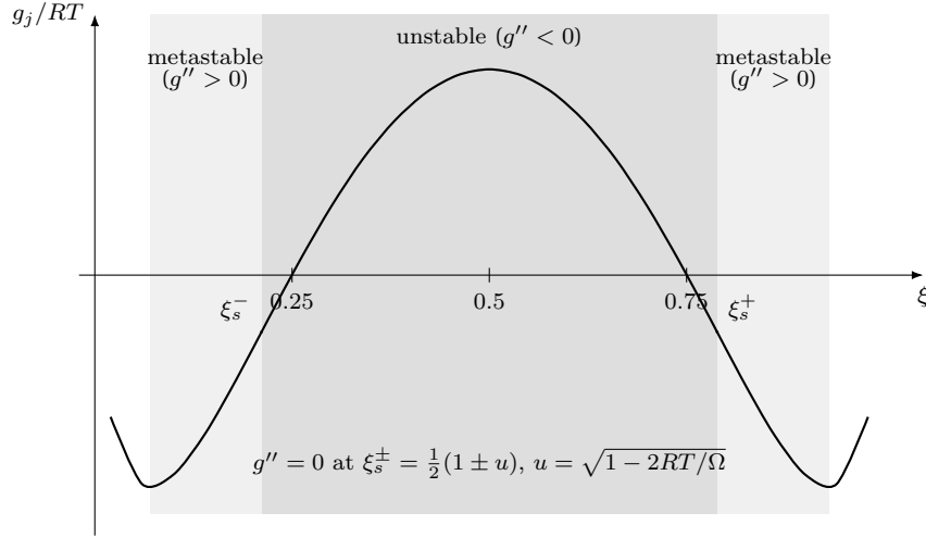
Figure 4: 자유에너지 g_j(\xi) 의 이중웰(신규, \Omega_j = 3RT ). 식 (1.9) 의 엔트로피 몫(아래로 볼록)과 \Omega 몫(가운데 위로)이 경쟁해 \Omega > 2RT 면 가운데가 언덕, 양쪽에 골 둘이 생긴다. 곡률 영점 g_j'' = 0 (식 (1.10)·(1.12))이 진한 띠(불안정)와 옅은 띠(준안정 — 핵생성 장벽, 히스테리시스 무대)의 경계 \xi_s^\pm 다. 이 두 점이 그림 3 전위 곡선의 두 극값이고, 그 전위 차가 \Delta U_j^{\text{hys}} (식 (1.16))다.
