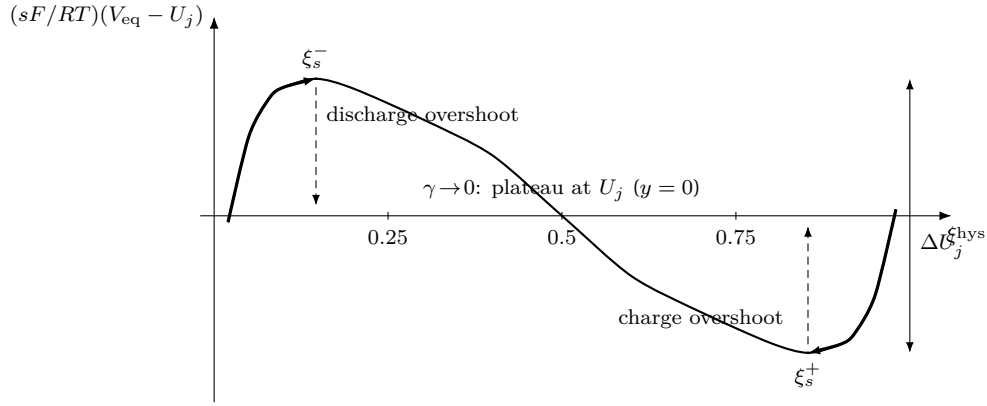
Figure 3: 비단조 평형 전위 V_{eq}(\xi)(\Omega_j = 4RT) 와 과주행. 방전(굵은 경로, 좌상)은 극대 \xi_s^- 까지, 충전(우하)은 극소 \xi_s^+ 까지 과주행해 중심이 갈라진다. 두 극값 차가 spinodal 상한 gap \Delta U_j^{\text{hys}} (식 (1.17)), 실측 분기는 \gamma_j 만큼 안쪽(식 (1.19)). \gamma \rightarrow 0 가역 한계에서 두 경로가 y = 0 plateau 로 합쳐진다.
