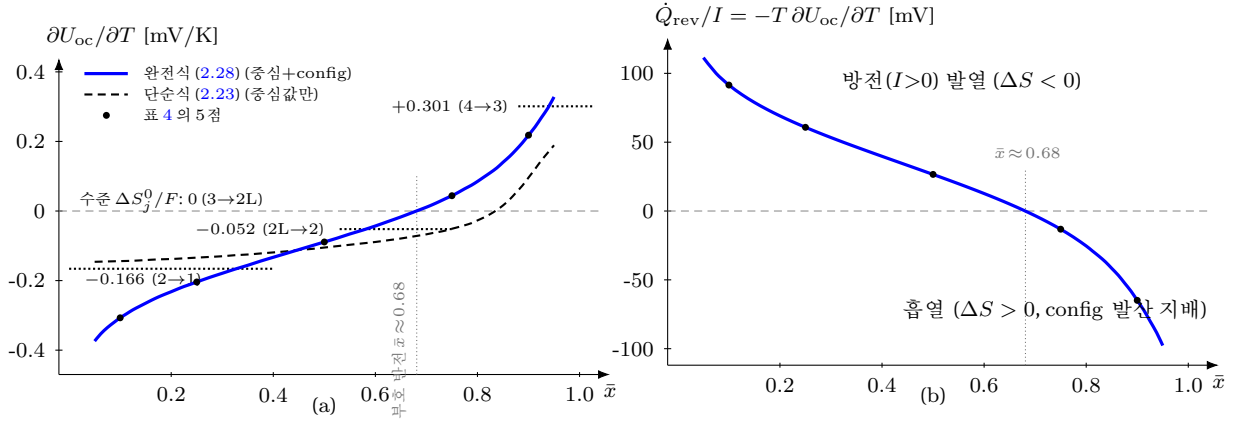
Figure 4: 완전식이 만드는 하프셀 엔트로피 계수와 가역 발열의 실제산 곡선 — 좌표는 식 그대로의 수치 평가다(4-전이 staging 입력: 표 1의 \Delta S_j^0 , w_j = RT/F(n_j=1) , 298.15 K; 각 \bar{x} 에서 전하 보존 음함수 (2.18)를 풀어 U_{oc} 를 얻은 뒤 평가). (a) \partial U_{oc}/\partial T(\bar{x}) — 파란 실선 = 완전식 (2.28)(중심 표준값+분포 config), 검은 파선 = 단순식 (2.23)(중심값만)이고 둘의 차가 봉우리 내부 config 항이다(파생 B). 점선 수평선은 전이별 수준 \Delta S_j^0/F — 곡선이 전이 경계마다 계단 없이 인접 수준 사이를 연속으로 지난다(파생 A의 연속 블렌드). ●는 표 4의 다섯 점과 일치하며 \bar{x}=0.25 값이 계산 예제 (§2.8.2)의 -0.204 (/단순식 -0.134 ) mV/K 다. (b) 가역 발열 \dot{Q}_{rev}/I = -T \partial U_{oc}/\partial T (식 (2.27)) — \bar{x} \approx 0.68 에서 방전 발열이 흡열로 스스로 반전한다(임의 함수·외부 스위치 없이 분포만으로). 완전식 곡선은 폭의 열적 서식 w_j = n_j RT/F 를 전제하며, 실측 폭이 T -동결에 가까우면 단순식이 보수적 기준이다 (§2.5.4).
