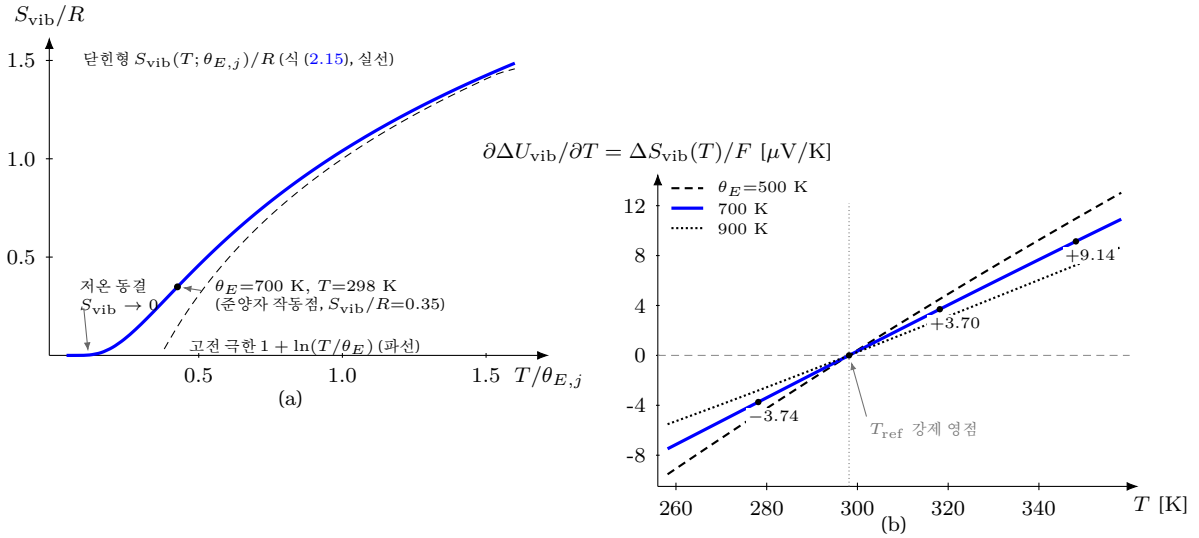
Figure 2: Einstein 진동 보정의 두 얼굴 — 좌표는 식 (2.15)·(2.17) 그대로의 수치 평가다. (a) 단원형 S_{\text{vib}}(T; \theta_{E,j})/R : 저온( u_j \rightarrow \infty )에서 0 으로 동결되고 고전 극한(파선) 1 + \ln(T/\theta_E) 에 T/\theta_E \gtrsim 1 에서 붙는다 — 앞 절이 중심 표준값에 흡수한 “ T -무관 상수”는 이 곡선을 T_{\text{ref}} 에서 한 번 평가해 동결한 값이다. ● 는 \theta_E = 700 \text{ K} \cdot 298 \text{ K} 의 준양자 작동점. (b) 중심 이동의 온도 기울기 \partial \Delta U_{\text{vib}} / \partial T = \Delta S_{\text{vib}}(T)/F : \theta_E = 500/700/900 \text{ K} 모두 T_{\text{ref}} 의 강제 영점을 지나 로그형 곡률로 자라며, ● 는 본문 §2.4.3 의 수치 ( \theta_E = 700 \text{ K} 에서 -3.74/0/+3.70/+9.14 \mu\text{V/K} ) 다. electronic 항( \propto T )은 이 강제 영점이 없어 두 함수형이 다운도 곡률 피팅에서 갈리고, 분리에는 준양자 창을 걸치는 온도점 셋 이상이 필요하다.
