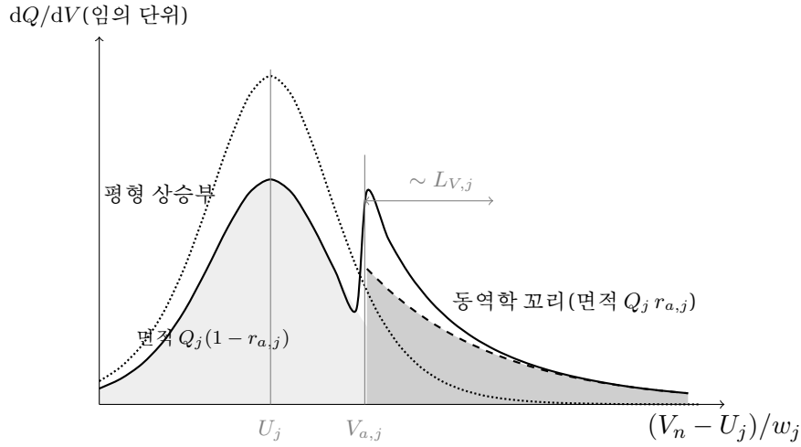
Figure 7: 단한식 (1.69) 한 전이의 해부( r_{a,j} = 0.315 , L_V = 3w ). 점선은 평형 중 (기준선), 파선은 동역학 꼬리, 실선이 단한식의 합이다. 상승부 실선이 점선보다 낮은 간격이 종 항의 (1 - r_{a,j}) 인자 — 꼬리로 넘어간 미완 몫의 회계 — 이고, 열은 음영(중 성분)과 진한 음영(꼬리 성분)의 면적이 각각 Q_j(1 - r_{a,j}) 와 Q_j r_{a,j} , 합이 정확히 Q_j 다(식 (1.70) 의 시각 짝). 꼬리는 V_{a,j} 에서 진폭 r_{a,j}/L_{V,j} 로 점화되어 단방향으로만 살며, 점화 계단은 지시함수의 모델 성질이라 r_{a,j} 가 클수록 크고 실측에서는 평형이 뭉개진다. 점화점이 U_j + 2.2w 에 놓인 것은 본 그림의 합성 조건에서 q -축 5% 컷이 맺히는 V -축 상(像)이라서다 — |dV/dq| 압축 때문에 V -축의 평형 중은 그 점에서 아직 유한하다.
