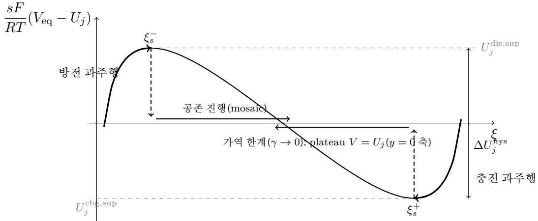
Figure 9: 비단조 평형 전위 (1.74) ( \Omega_j = 4RT )와 과주행 경로 — 극값이 spinodal 에 서는 근거는 식 (1.75). 방전(굵은 경로, 좌상)은 상승 준안정 가지를 타고 극대 \xi_s^- 까지 과주행한 뒤, 분리가 점화되며 공존 plateau ( V = U_j, y = 0 축)로 낙하해(점선 화살표) mosaic 공존으로 진행한다. 충전(우하)은 거울상으로 극소 \xi_s^+ 까지 과주행한다. 두 극값의 차가 spinodal 상한 gap \Delta U_j^{\text{hys}} 이고(위첨자 sup는 spinodal 상한 표시), 실측 분기는 축소 인자 \gamma_j 만큼 그 안쪽에 선다 — \gamma \rightarrow 0 의 가역 한계에서 두 경로가 모두 y = 0 의 plateau 로 합쳐진다.
