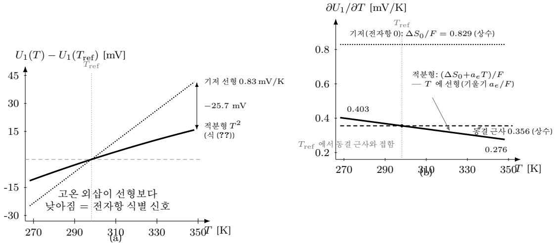
Figure 3: T1 전이 중심의 온도 함수형이 갖는 전자항 식별 신호 — 좌표는 식 (??) 그대로의 수치 평가다( \Delta S_0 = +80 J/(mol K) 대표 스케일[tier B — §??], 게이트 중심의 몰당 단원식(식 (??)·(??)) 에서 a_e = -0.153 J/(mol K 2 ), T_{ref} = 298.15 K). (a) U_1(T) : 전자항이 없으면 기저 선형(점선, 0.83 mV/K), 전자항( \propto T )을 적분하면 T^2 곡률(실선) — a_e < 0 라 고온 외삽이 선형 외삽보다 낮아지고 (348 K 에서 -25.7 mV) 이것이 다운도 피팅의 식별 신호다. (b) 같은 내용의 기울기 공간: \partial U_1 / \partial T = (\Delta S_0 + a_e T)/F 가 T 에 선형으로 감소한다( 0.403 \rightarrow 0.276 mV/K). 현행 동결 근사(파선 — \Delta S_e 를 T_{ref} 상수로 두는 §?? 의 단일-기준 근사)는 적분형의 T_{ref} 접선이라 (a)에서는 실선과 (a_e/2F)(T - T_{ref})^2 (348 K 에서 -2.0 mV) 만큼만 이차로 벌어지고, (b)의 기울기 공간에서 상수 대 선형으로 명확히 갈린다.
