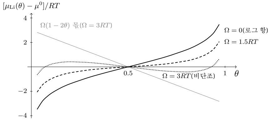
Figure 3: 화학퍼텐셜 (1.13) 의 해부(실계산). 실선은 \Omega = 0 의 로그(섞임 엔트로피) 몫 — 채울수록 값어치가 단조로 오른다. 회색 가는 선은 상호작용 몫 \Omega(1 - 2\theta) ( \Omega = 3RT ) — 반대 기울기의 직선이다. 로그 몫에 각자의 \Omega(1 - 2\theta) 를 더하면: \Omega = 1.5RT (파선)는 가운데가 평평해진 단조 곡선, \Omega = 3RT > 2RT (점선)는 비단조 — 한 값어치에 세 조성이 대응하며, 이것이 상분리의 씨앗이다 (§1.5).
