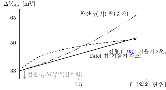
Figure 14: 관측 gap 의 분해 (1.93) (실계산: 절편 33 mV, 기울기 20 mV/단위). 실선이 가산 분해의 예측 — |I| \rightarrow 0 절편이 열역학 같림, 기울기가 분극이다. 파선은 charge-transfer 의 Tafel 휨(기울기 점감), 점선은 확산 한계· \gamma_j(|I|) 의 휨(점증) — 두 휨이 가산 분해 전제의 위반 지문이며 진단표 (§1.15)가 받는다.
