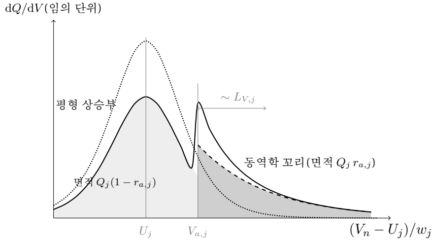
Figure 11: 닫힌식 (1.79) 한 전이의 해부( r_{a,j} = 0.315 , L_V = 3w ). 점선은 평형 중 (기준선), 파선은 동역학 꼬리, 실선이 닫힌식의 합이다. 상승부 실선이 점선보다 낮은 간격이 종 항의 (1 - r_{a,j}) 인자 — 꼬리로 넘어간 미완 몫의 회계 — 이고, 열은 음영(중 성분)과 진한 음영(꼬리 성분)의 면적이 각각 Q_j(1 - r_{a,j}) 와 Q_j r_{a,j} , 합이 정확히 Q_j 다(식 (1.80) 의 시각 짝). 꼬리는 V_{a,j} 에서 진폭 r_{a,j}/L_{V,j} 로 점화되어 단방향으로만 살며, 점화 계단은 지시함수의 모델 성질이라 r_{a,j} 가 클수록 크고 실측에서는 평활이 뭉갸다. 점화점 U_j + 2.25w 는 꼬리 형상이 한눈에 들어오도록 잡은 예시 배치다 — 실데이터의 V_{a,j} 는 컷 정의 (§1.15 (3')) 가 그 조건의 측정 V_n(q) 위에서 정하며, 보통 종의 더 깊은 어깨에 맺힌다.
