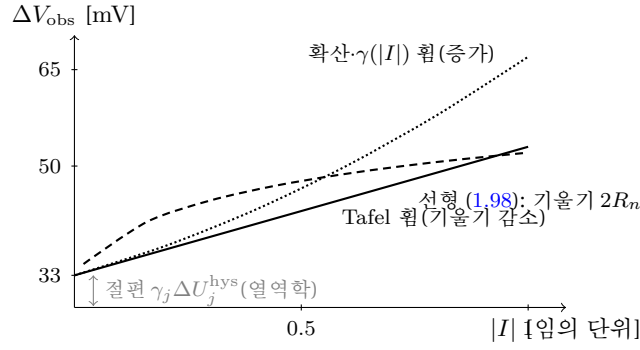
Figure 14: 관측 gap 의 분해 (1.98) (실계산: 절편 33 mV, 기울기 20 mV/단위). 실선이 가산 분해 — |I| \rightarrow 0 절편이 열역학, 기울기가 분극. 파선은 charge-transfer Tafel 휨 (점감), 점선은 확산· \gamma_j(|I|) 휨 (점증) — 두 휨이 가산 분해 위반 지문이며 진단표 (§1.15)가 받는다.
