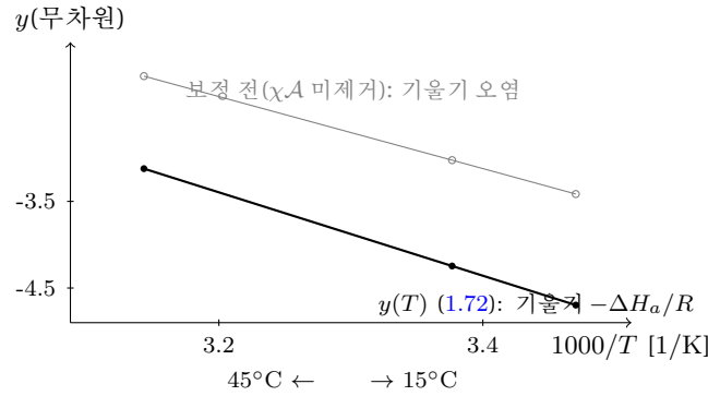
Figure 9: Arrhenius 회귀 (1.73) ( \Delta H_a = 40 kJ/mol, 절편 12, 세 온도 15/23/45°C). 검정: 보정된 y(T) (1.72) — 1/T 선형, 기울기 -\Delta H_a/R . 회색: 구동항 \chi A_j/RT 미제거 — offset 이 온도마다 달라 기올기 오염. S4 가 \chi 를 먼저 닫는 이유 (§1.15).
