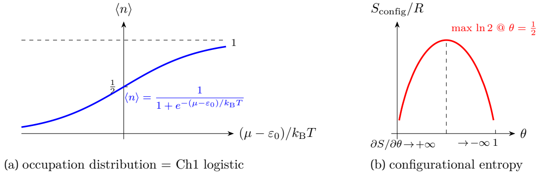
Figure 19: (a) 단일 자리 점유 분포 \langle n \rangle (1.98) — Fermi-Dirac 와 동형이며 Chapter 1 logistic 평형 점유의 기원. (b) configurational 엔트로피 S_{\text{config}}(\theta) (1.105); 중심 \theta = \frac{1}{2} 에서 최대 \ln 2 , 부분물 \partial S_{\text{config}}/\partial \theta = -R \ln[\theta/(1-\theta)] 가 양 끝에서 \pm\infty 로 발산(봉우리 내부 \partial U_{\text{oc}}/\partial T 의 분포 항).
