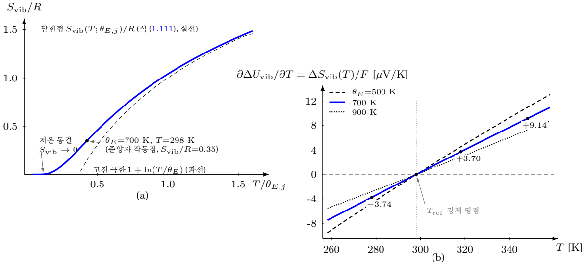
Figure 20: Einstein 진동 보정의 두 얼굴 — 좌표는 식 (1.111)·(1.113) 그대로의 수치 평가다. (a) 단한형 S_{\text{vib}}(T; \theta_{E,j})/R : 저온( u_j \rightarrow \infty )에서 0 으로 동결되고 고전 극한(파선) 1 + \ln(T/\theta_E) 에 T/\theta_E \gtrsim 1 에서 붙는다 — 앞 절이 중심 표준값에 흡수한 “ T -무관 상수”는 이 곡선을 T_{\text{ref}} 에서 한 번 평가해 동결한 값이다. ● 는 \theta_E = 700 \text{ K} · 298 \text{ K} 의 준양자 작동점. (b) 중심 이동의 온도 기울기 \partial \Delta U_{\text{vib}} / \partial T = \Delta S_{\text{vib}}(T)/F : \theta_E = 500/700/900 \text{ K} 모두 T_{\text{ref}} 의 강제 영점을 지나 로그형 곡률로 자라며, ● 는 본문 §1.14.3 의 수치 ( \theta_E = 700 \text{ K} 에서 -3.74/0/+3.70/+9.14 \mu\text{V/K} ) 다. electronic 항( \propto T )은 이 강제 영점이 없어 두 함수형이 다운도 곡률 피팅에서 갈리고, 분리에는 준양자 창을 걸치는 온도점 셋 이상이 필요하다.
