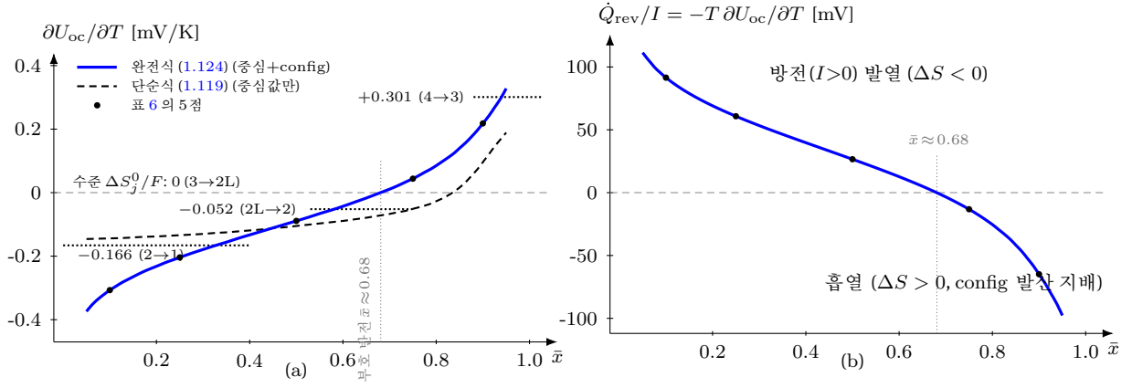
Figure 22: 완전식이 만드는 하프셀 엔트로피 계수와 가역 발열의 실제산 곡선 — 좌표는 식 그대로의 수치 평가다(4-전이 staging 입력: 표 3의 \Delta S_j^0 , w_j=RT/F(n_j=1) , 298.15 K; 각 \bar{x} 에서 전하 보존 음함수 (1.114)를 풀어 U_{oc} 를 얻은 뒤 평가). (a) \partial U_{oc}/\partial T(\bar{x}) — 파란 실선 = 완전식 (1.124)(중심 표준값+분포 config), 검은 파선 = 단순식 (1.119)(중심값만)이고 둘의 차가 봉우리 내부 config 항이다(파생 B). 점선 수평선은 전이별 수준 \Delta S_j^0/F — 곡선이 전이 경계마다 계단 없이 인접 수준 사이를 연속으로 지난다(파생 A의 연속 블렌드). ●는 표 6의 다섯 점과 일치하며 \bar{x}=0.25 값이 계산 예제 (§1.18.2)의 -0.204 (/단순식 -0.134 ) mV/K 다. (b) 가역 발열 \dot{Q}_{rev}/I = -T \partial U_{oc}/\partial T (식 (1.123)) — \bar{x} \approx 0.68 에서 방전 발열이 흡열로 스스로 반전한다(임의 함수·외부 스위치 없이 분포만므로). 완전식 곡선은 폭의 열적 서식 w_j=n_jRT/F 를 전제하며, 실측 폭이 T -동결에 가까우면 단순식이 보수적 기준이다 (§1.15.4).
