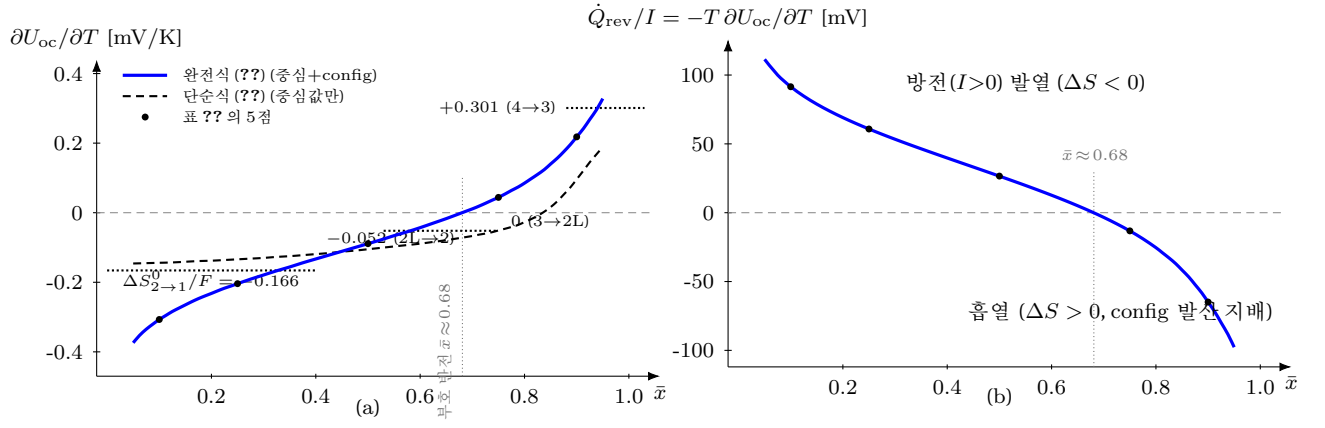
Figure 1: 완전식이 만드는 하프셀 엔트로피 계수와 가역 발열의 실제산곡선 — 좌표는 식 그대로의 수치 평가다(4 전이 staging 입력: 표 ?? 의 \Delta S_j^0 , w_j=RT/F(n_j=1) , 298.15 K; 각 \bar{x} 에서 전하 보존 음함수 (??) 를 풀어 U_{oc} 를 얻은 뒤 평가). (a) \partial U_{oc}/\partial T(\bar{x}) — 파란 실선 = 완전식 (??)(중심 표준값+분포 config), 검은 파선 = 단순식 (??)(중심값만) 이고 둘의 차가 봉우리 내부 config 향이다(파생 B). 점선 수평선은 전이별 수준 \Delta S_j^0/F — 곡선이 전이 경계마다 계단 없이 인접 수준 사이를 연속으로 지난다(파생 A 의 연속 블렌드). ● 는 표 ?? 의 다섯 점과 일치하며 \bar{x}=0.25 값이 계산 예제 (§??) 의 -0.204 /(단순식 -0.134 ) mV/K 다. (b) 가역 발열 \dot{Q}_{rev}/I = -T \partial U_{oc}/\partial T (식 (??)) — \bar{x} \approx 0.68 에서 방전 발열이 흡열로 스스로 반전한다(임의 함수·외부 스위치 없이 분포만으로). 완전식 곡선은 폭의 열적 서식 w_j=n_j RT/F 를 전제하며, 실측 폭이 T -동결에 가까우면 단순식이 보수적 기준이다 (§??).
