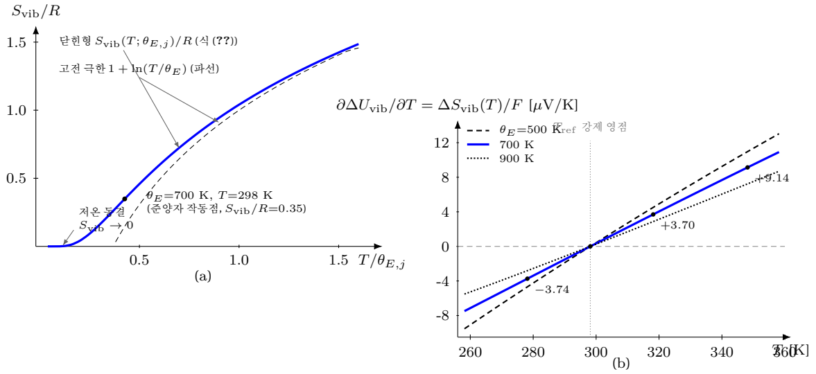
Figure 2: Einstein 진동 보정의 두 얼굴 — 좌표는 식 (??)·(??) 그대로의 수치 평가다. (a) 단진형 S_{\text{vib}}(T; \theta_{E,j})/R : 저온( u_j \rightarrow \infty )에서 0 으로 동결되고 고전 극한(파선) 1 + \ln(T/\theta_E) 에 T/\theta_E \gtrsim 1 에서 붙는다 — 앞 절이 중심 표준값에 흡수한 “ T -무관 상수”는 이 곡선을 T_{\text{ref}} 에서 한번 평가해 동결한 값이다. ● 는 \theta_E = 700 \text{ K} \cdot 298 \text{ K} 의 준양자 작동점. (b) 중심 이동의 온도 기울기 \partial \Delta U_{\text{vib}} / \partial T = \Delta S_{\text{vib}}(T)/F : \theta_E = 500/700/900 \text{ K} 모두 T_{\text{ref}} 의 강제 영점을 지나 로그형 곡물로 자라며, ● 는 본문 §?? 의 수치 ( \theta_E = 700 \text{ K} 에서 -3.74/0/+3.70/+9.14 \mu\text{V/K} ) 다. electronic 항( \propto T )은 이 강제 영점이 없어 두 함수형이 다운도 곡률 피팅에서 갈리고, 분리에는 준양자 창을 걸치는 온도점 셋 이상이 필요하다.
