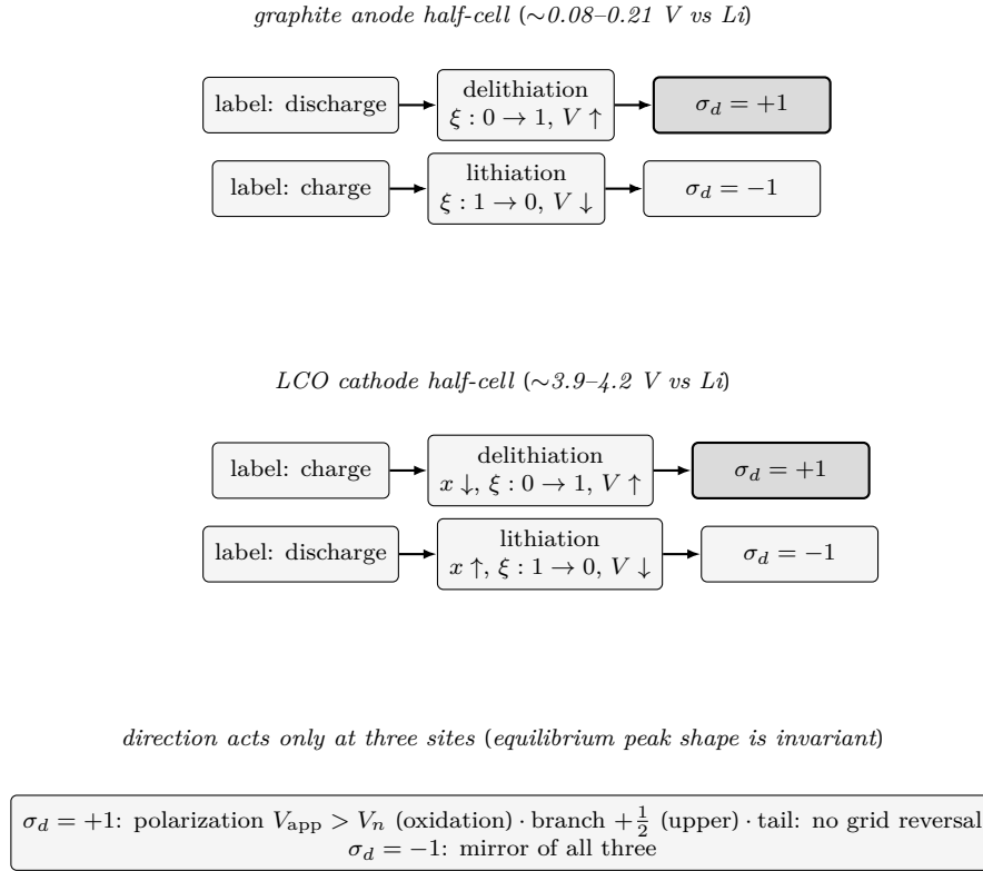
Figure 15: 충·방전 라벨과 탈리튬화 방향의 대응(신규 그림). \sigma_d 슬롯의 물리 내용은 셀 라벨이 아니라 “작동 전극의 탈리튬화 = +1”(식 (1.73))이다 — 흑연 하프셀은 방전이, LCO 하프셀은 충전이 \sigma_d = +1 슬롯(음영 상자)에 간다. 방향은 분극·분기·꼬리 세 작용처에만 작용하고 평형 종은 \xi \leftrightarrow 1 - \xi 교환에 불변이다.
