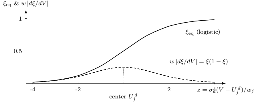
Figure 11: 평형 진행률과 그 미분(v7-11 유래). 실선 = \xi_{eq} logistic(식 (1.53)), 파선 = 폭으로 규격화한 미분 w_j|d\xi_{eq}/dV| = \xi_{eq}(1 - \xi_{eq}) - z = 0 (중심 U_j^d )에서 최대 \frac{1}{4} 인 종 모양. 이 종이 다음 절의 평형 peak 이고, 방향에 불변(양수)이다.
