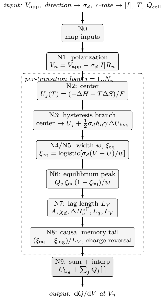
Figure 1: 한 곡선을 그리는 코드 진행(spine). 외부 실험조건이 curve facade 에서 (\sigma_d, |I|, T, Q_{cell}) 로 환산(N0)되어 코어 dqdv 로 들어가고, 분극으로 내부 전위 V_n 을 얻은 뒤(N1), 전이 j 마다 평형 중심·히스 분기·폭·평형 진행률·평형 peak·지연 길이·인과 꼬리를 계산해(N2–N8) 합산·역보간한다(N9). 본 문건의 절 순서가 이 노드 순서를 따른다(통계역학 기초 Part 0 은 N0 뒤에 삽입된 기초 절). 파선 상자가 코드의 전이 루프(for tr in transitions). 그림 출처 — v7-11 의 spine 그림을 그대로 채택했다.
