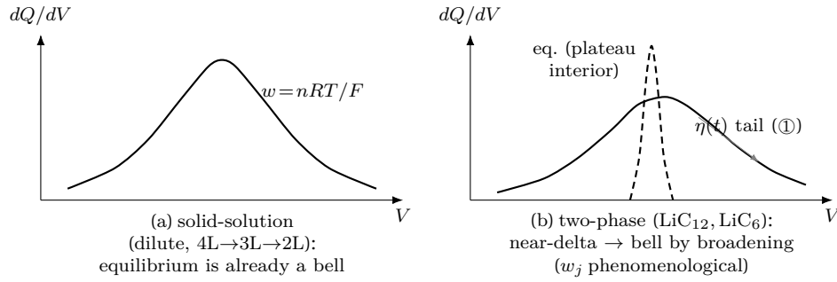
Figure 12: 평형 모양과 broadening(신규). (a) 연속 고용체 전이 — 평형 단일 입자 dQ/dV 가 이미 폭 n_j RT/F 의 종(식 (1.55)), broadening 불요. (b) 두-상 전이 — 평형은 plateau 내부에서 거의 날카로운 선(파선; 양끝 단상 꼬리 탓에 폭이 정확히 0 은 아님) 이고, 실측은 세 출처가 펼친 치우친 종(실선) 이다: ① 유한율속 비대칭 꼬리 (§1.8–§1.9 의 L_V , |I| \rightarrow 0 소멸), ② 전류 무관한 가장자리 내재 폭 ( \sim RT/F ), ③ 겉보기 중심 U_{app} = U_j + \eta 의 입자간 \eta 산포를 forward 평균한 앙상블 뭉(식 (1.56)). ①의 \eta(t) (한 입자의 시간 변화)와 ③의 입자간 \eta 산포는 같은 과전압의 다른 평균이며, 평형 중심 U_j 는 입자 무관 상수다 — 분포하는 것은 \eta . 세 출처의 지위와 한정(폭 w_j 의 현상학적 지위·흑연 두-상 국한· \rho(U_{app}) 역산 금지·사이즈 배제)은 본문 (b)·(c).
