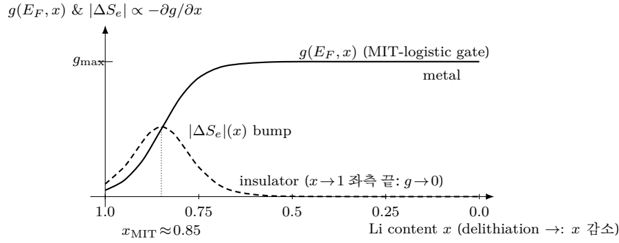
Figure 16: LCO 전자 엔트로피의 MIT-logistic 게이트(신규). 실선 = g(E_F, x) (식 (1.92)): x \approx 1 절연체에서 \approx 0 , 탈리튬화로 x_{\text{MIT}} \approx 0.85 부근에서 metal 의 g_{\text{max}} = 13 \text{ e/eV/atom} 으로 커진다. 파선 = 탈리튬화 시 방출되는 부분물 전자 엔트로피 |\Delta S_e| = -\partial S_e / \partial x \propto -\partial g / \partial x > 0 (식 (1.88)·단편식 (1.93); 삽입 기준 \Delta S_e = \partial S_e / \partial x < 0 의 절댓값으로, x_{\text{MIT}} 에서 \sigma(1-\sigma) 가 최대): 전이 중심의 국소 봉우리다 — 작지만(게이트골 몰당 \approx -46 \text{ J/(mol K)} , §1.11.6.3) MIT 구간에만 켜지는 게이트라 config 단독으로 대체 불가. \Delta S_{e,j} \propto T 라 다른 항과 달리 전자 기여의 \partial U / \partial T 가 T 에 선형(§1.11.6.2; U-이동은 \propto T^2 ). 흑연엔 이 봉우리가 없다( g(E_F) 변화 미미).
