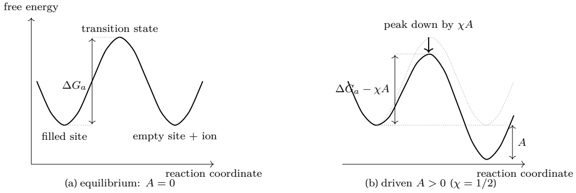
Figure 9: 활성화 장벽 그림(신규). (a) 평형 — 두 골짜기 같은 높이, 속도는 Eyring 식. (b) 구동력 \mathcal{A}_j 가 도착 골짜기를 내리면 정방향 장벽 \Delta G_a - \chi \mathcal{A} , 역방향 \Delta G_a + (1 - \chi)\mathcal{A} 로 비대칭 이동 (식 (1.50); 두 속도의 비가 식 (1.51) detailed balance). 점선은 (a). 온도는 분모 RT 로 진입. 이 그림이 식 (1.53) logistic 과 §1.8의 L_q 두 결과의 공통 출발점이다.
