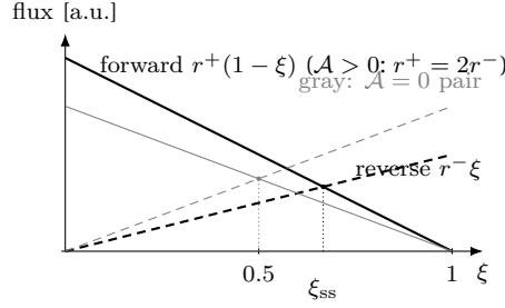
Figure 5: 정지점 (1.29): 정방향 r^+(1-\xi) (감소 직선)과 역방향 r^-\xi (증가 직선)의 교점(신규). \mathcal{A} > 0 ( r^+ = 2r^- , 검정)이면 \xi_{ss} = 2/3 , \mathcal{A} = 0 (회색)이면 \frac{1}{2} — 이 교점이 식 (1.30) logistic 으로 닫힌다.
